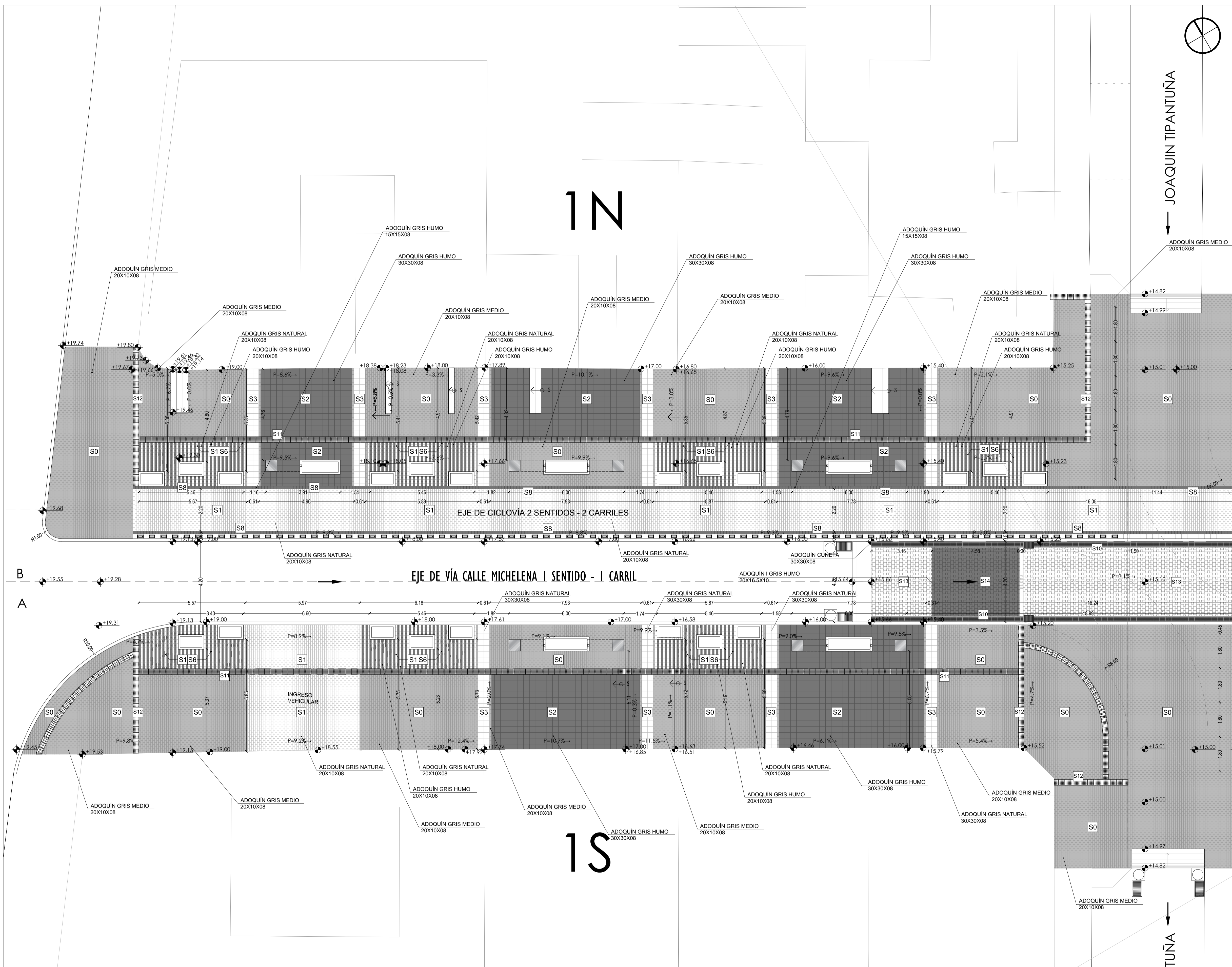
PLANTA DE PISOS PASEO PEATONAL LA MICHELINA MANZANA 1 ESC 1:100
