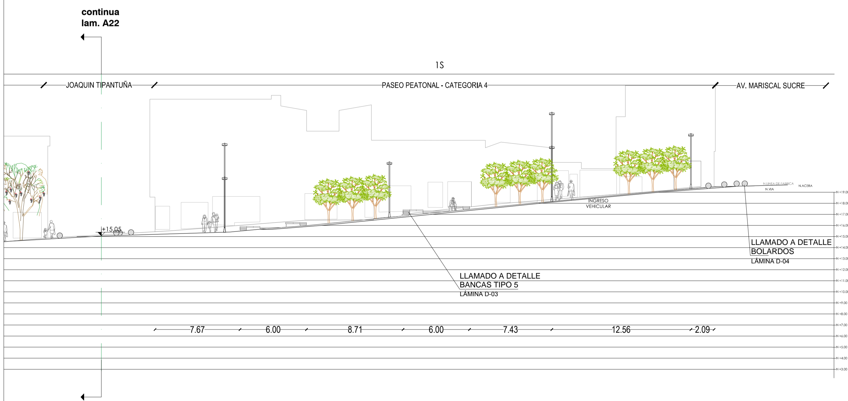
CORTE A - A` ESC 1:200
