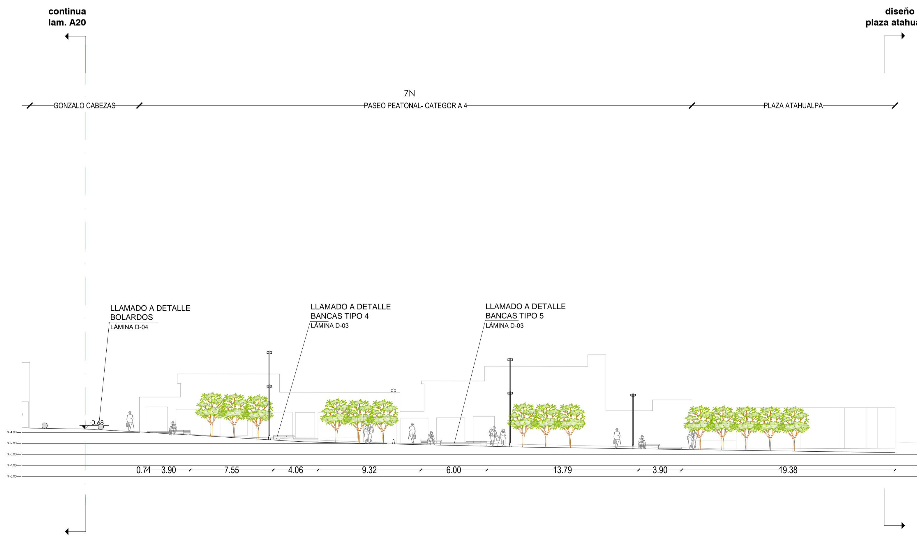
CORTE B - B` ESC 1:200
