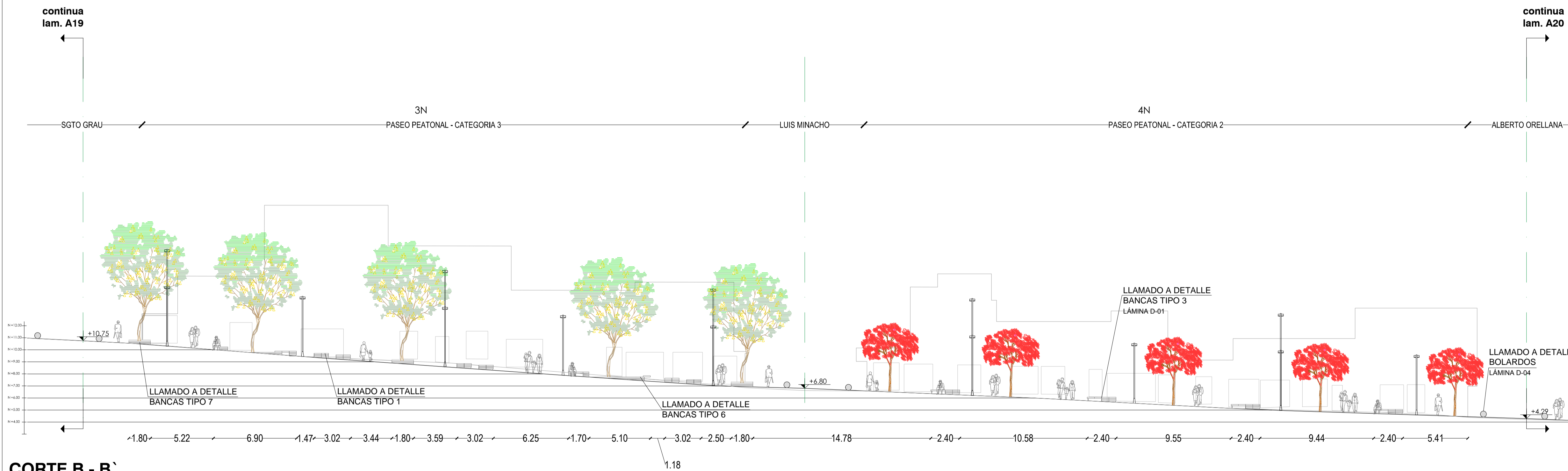
CORTE B - B` ESC 1:200
