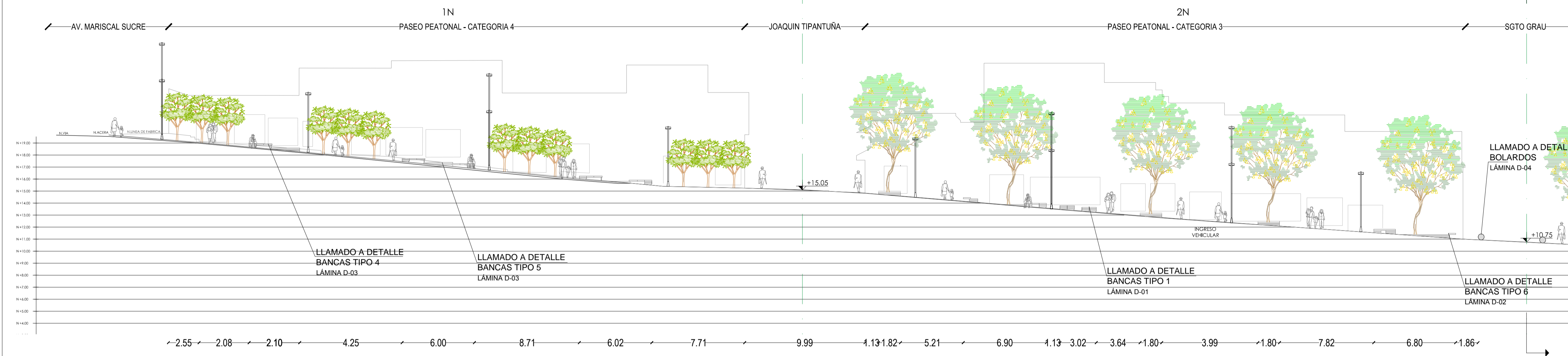
CORTE B - B` ESC 1:200
