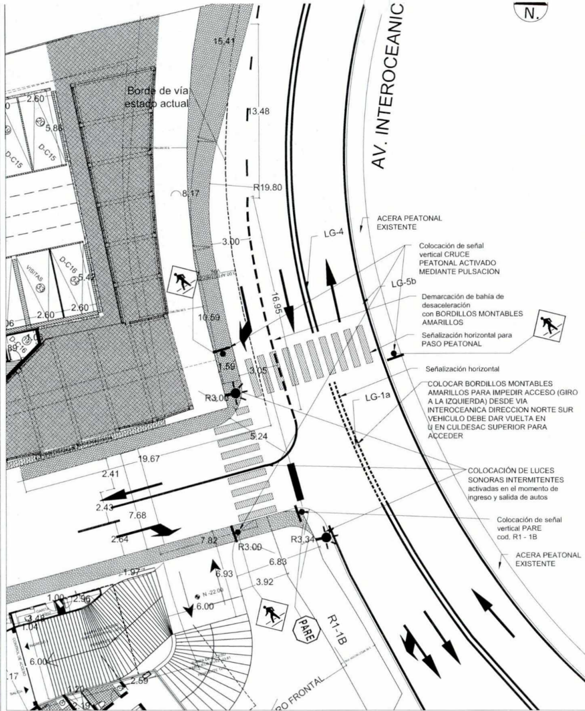
DETALLE DE ACCESO Esc: 100
