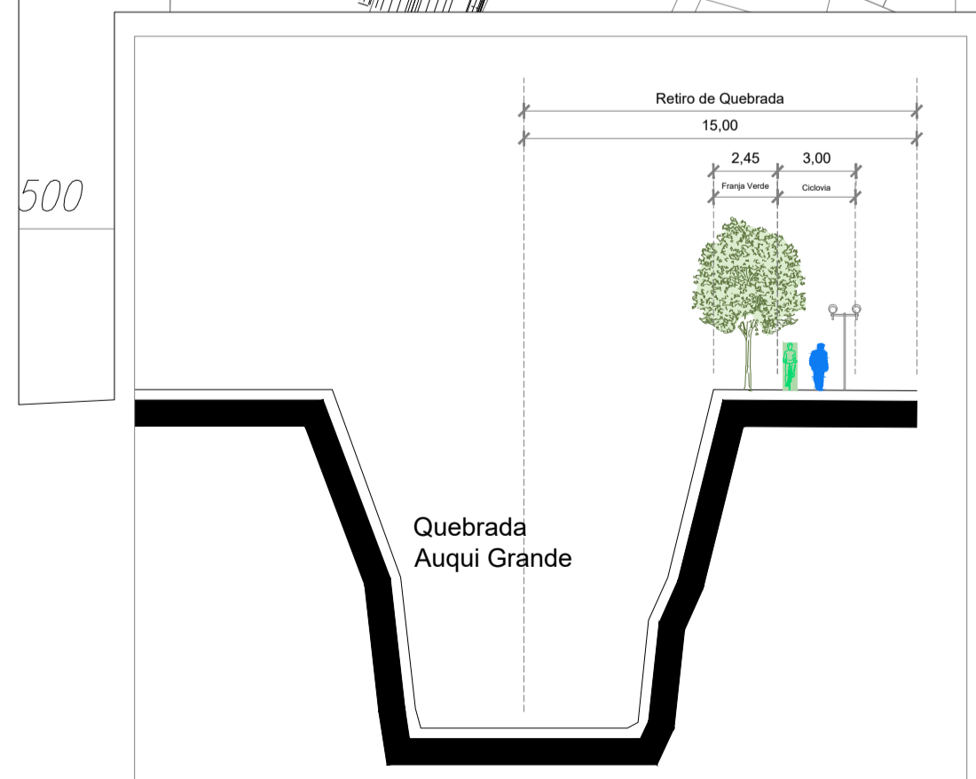
CORTE EN BORDE DE QUEBRADA esc 1:250
