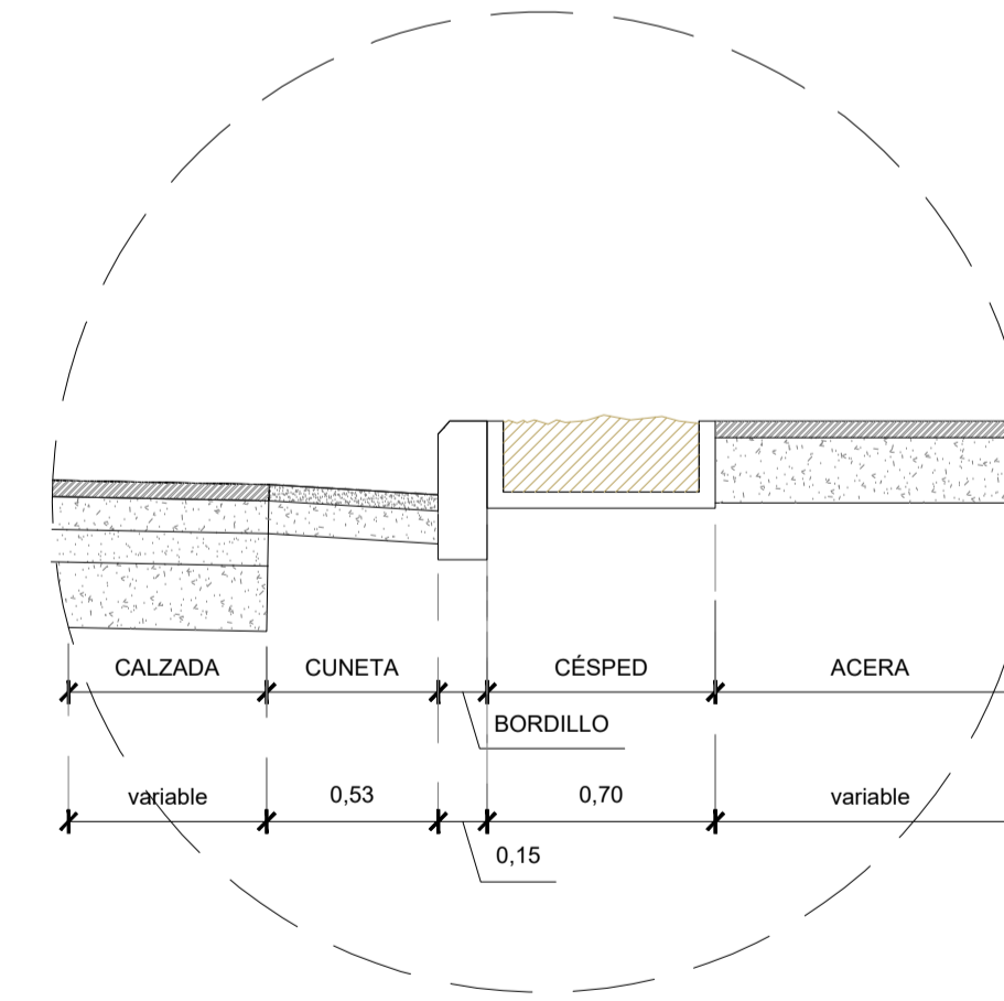
DETALLE 3 Encuentro Borde de Acera (sin ciclovia) + suelo permeable y Calzada escala 1.25
