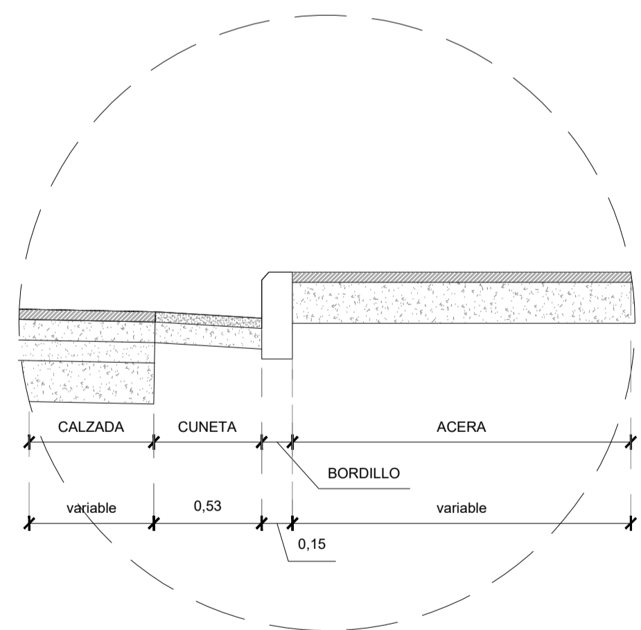
DETALLE 1 Encuentro Borde de Acera sin vegetación y Calzada escala 1.25
