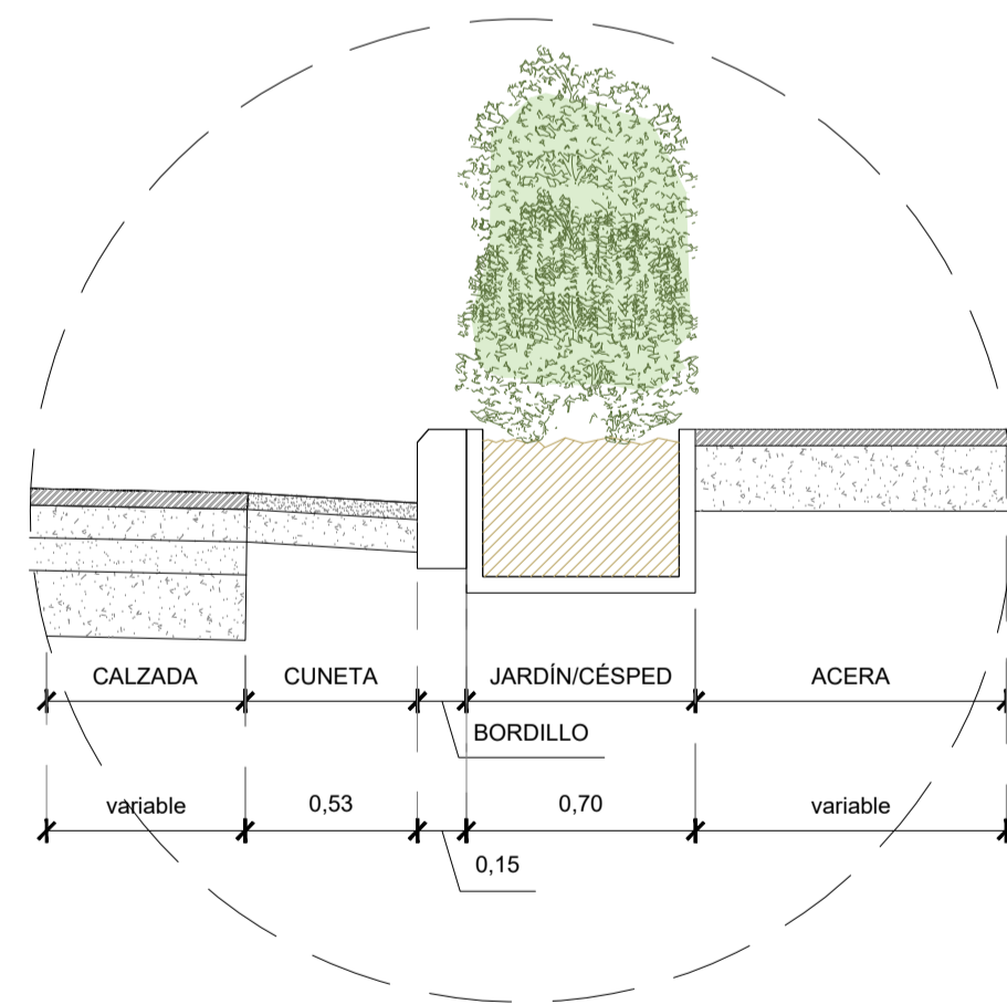
DETALLE 2 Encuentro Borde de Acera con vegetación + suelo permeable y Calzada escala 1.25
