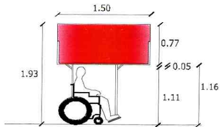
VISTA LATERAL.
