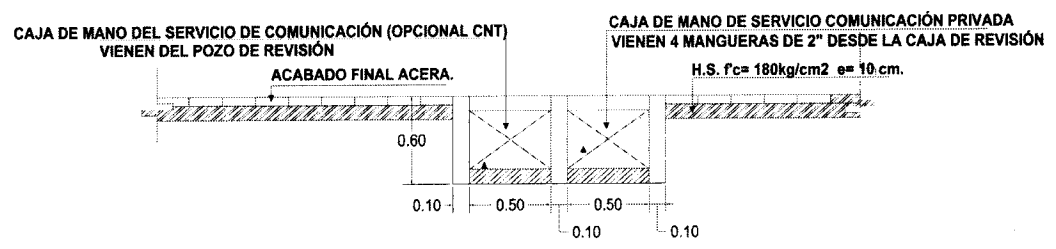
CORTE B-B'
