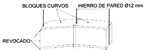
DETALLE BLOQUES CURVOS
