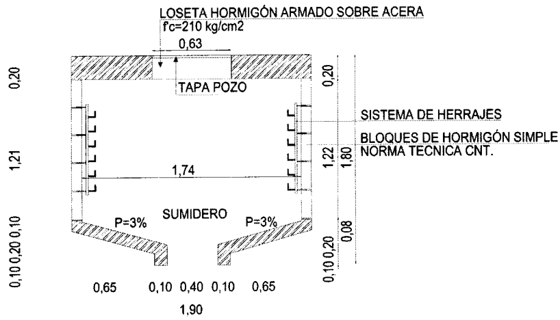
CORTE TRANSVERSAL
