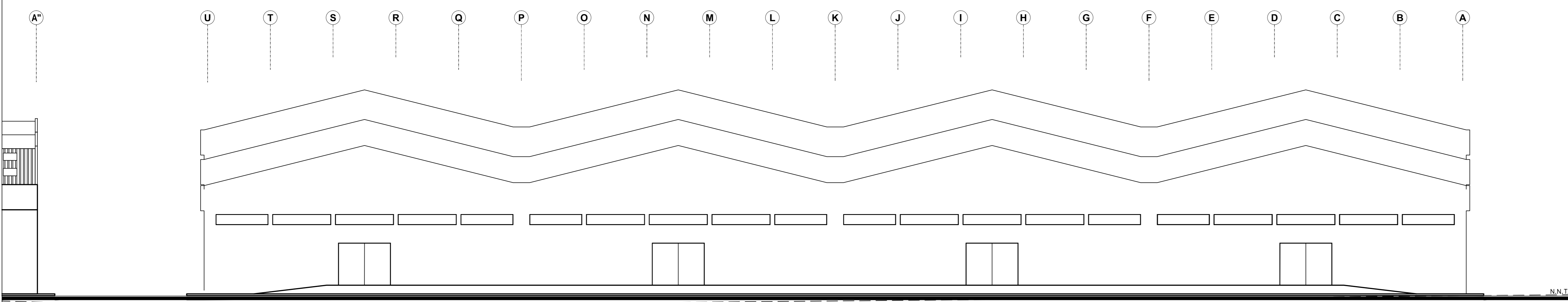
ELEVACIÓN OCCIDENTAL BODEGAS 9-12 ESCALA 1:200
