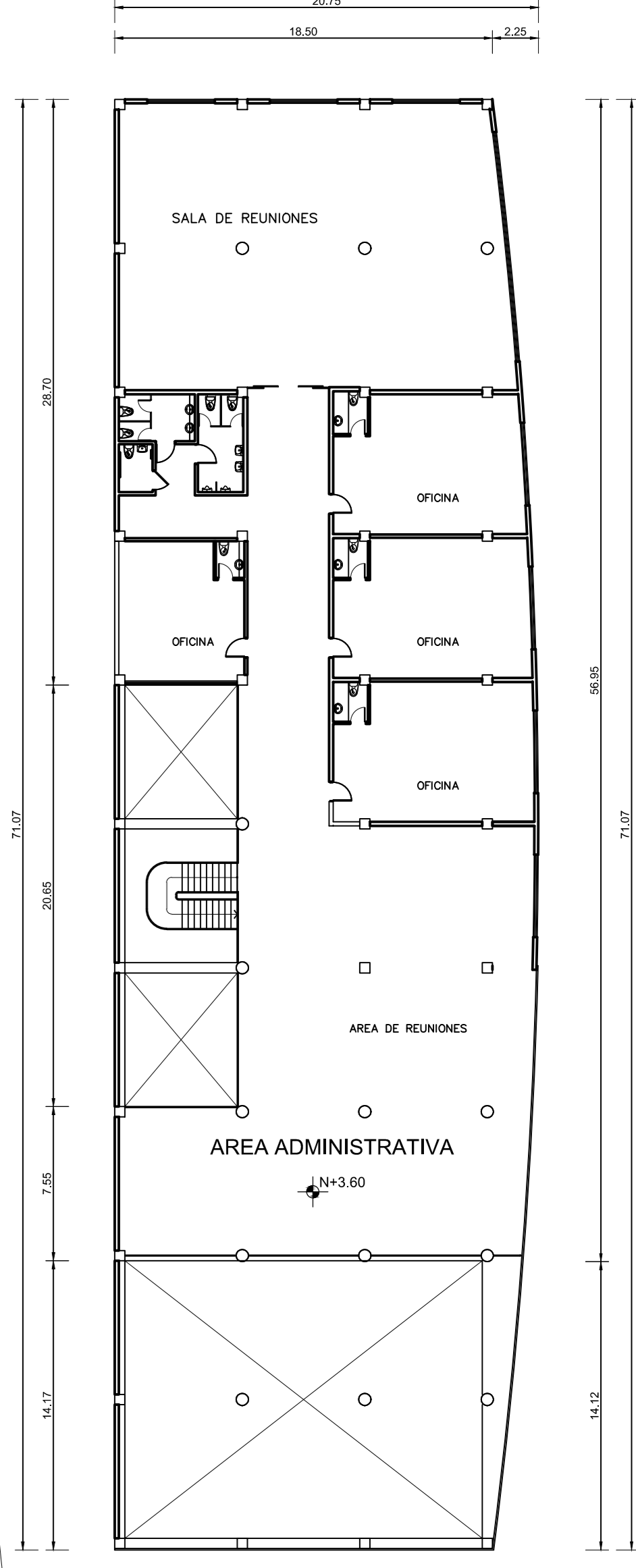
PLANTA ALTA AREA ADMINISTRATIVA ESCALA: 1:100
