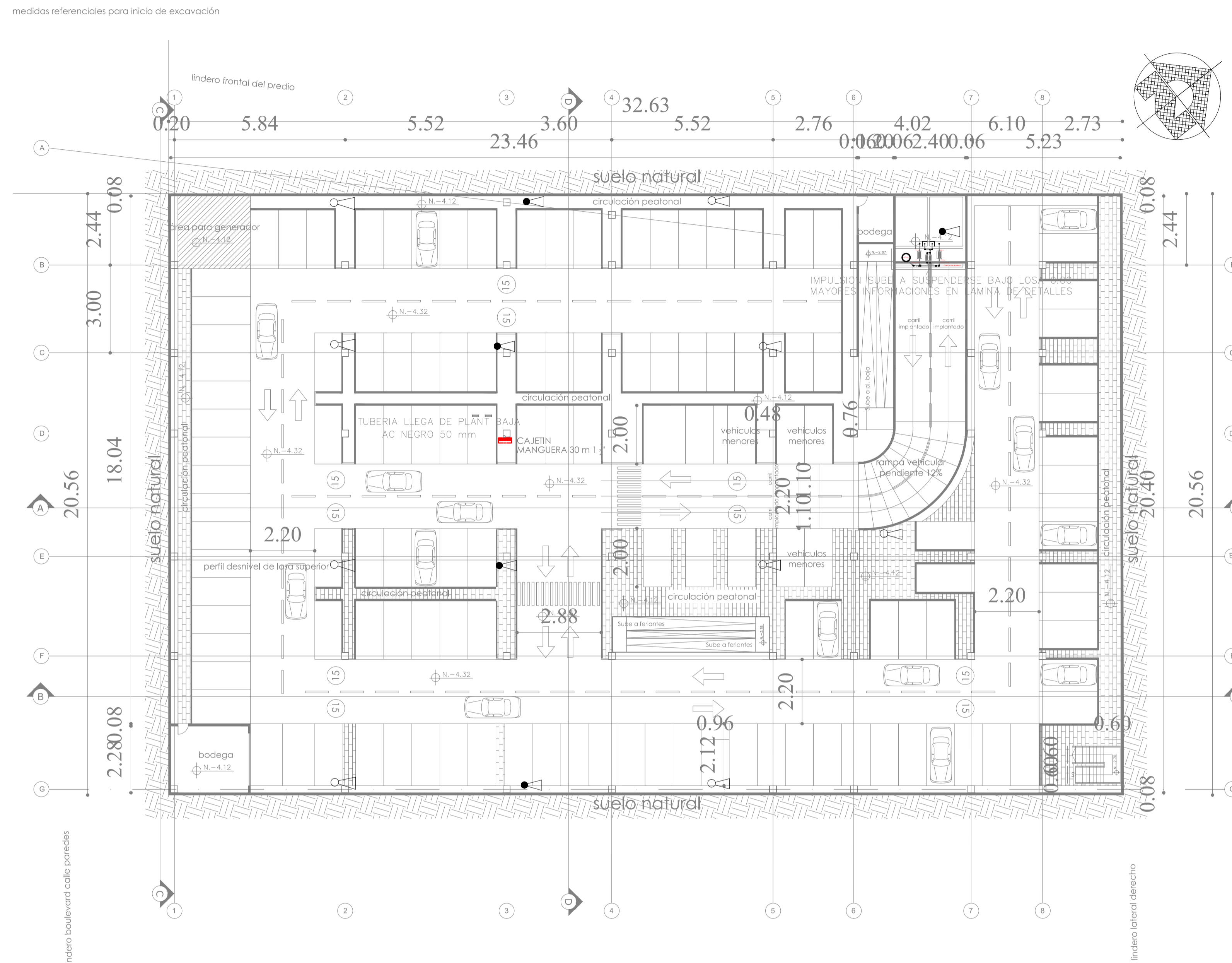
PLANTA SUBSUELO. N.- 4.32 1-250
