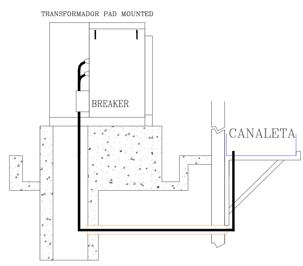
CORTE C-D ESC: 1:25
