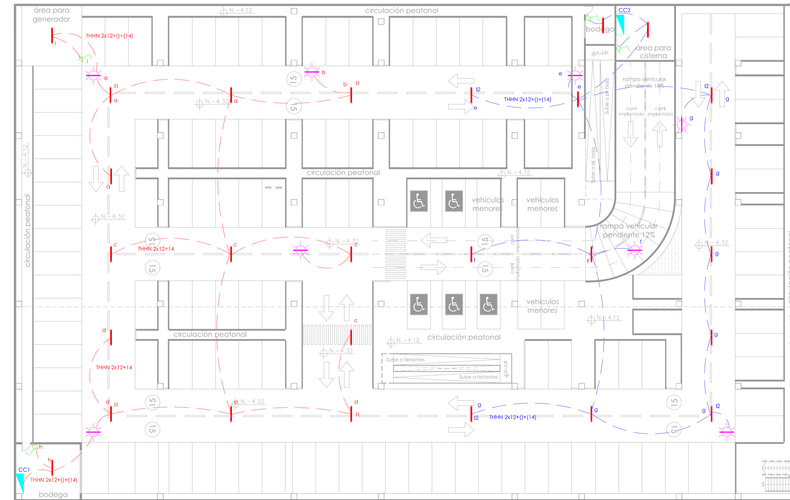
PLANTA SUBSUELO N -4.32 Esc 1:200
