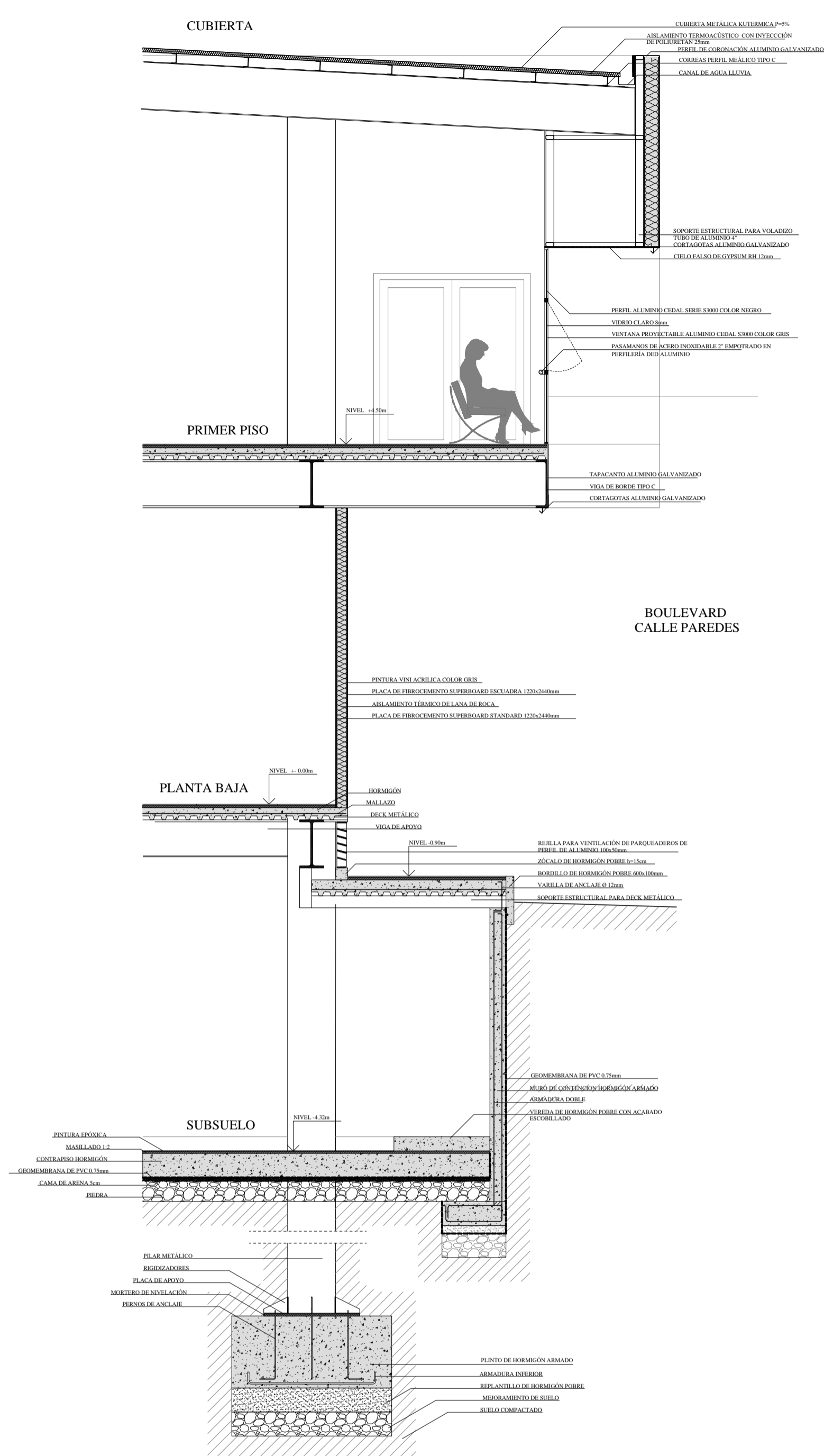
CORTE POR MURO FACHADA BOULEVARD ESC: 1-50
