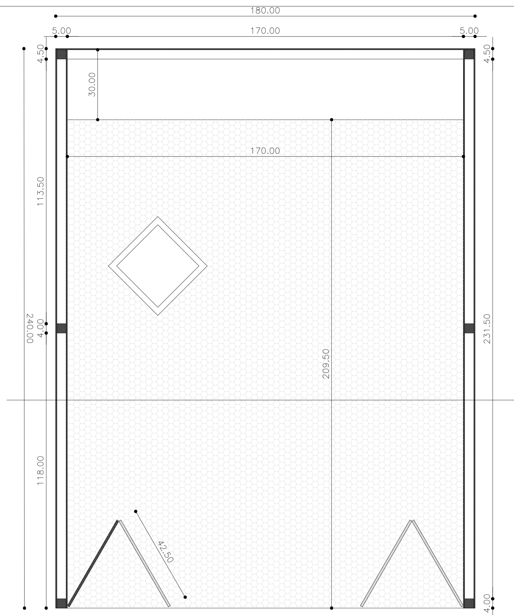
PLANTA ESC: 1-10
