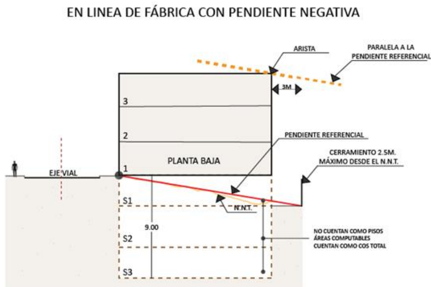
Gráfico 2.021 En línea de Fábrica con Pendiente Negativa
