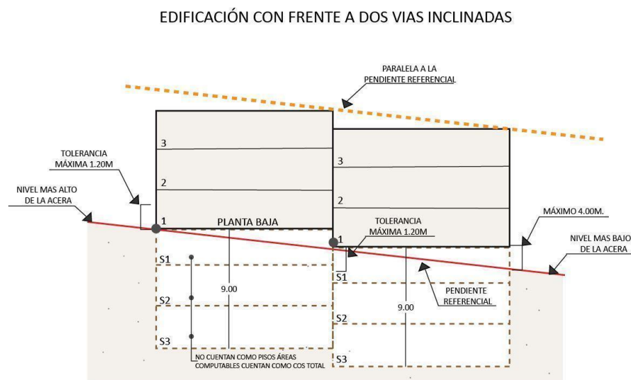
Gráfico 2.030 Edificación con Frente a Dos Vías Incluidas - Corte
