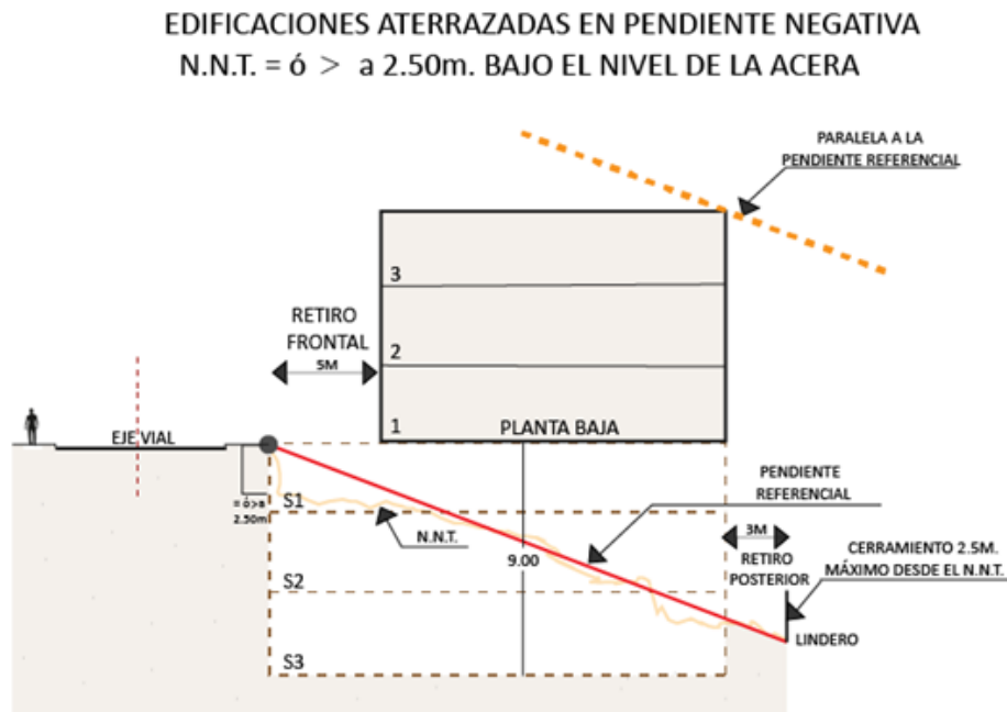
Gráfico 2.029 Edificaciones Aterrazadas con Retiro Frontal y Pendiente Negativa N.N.T. \geq 2.50m bajo el nivel de acera
