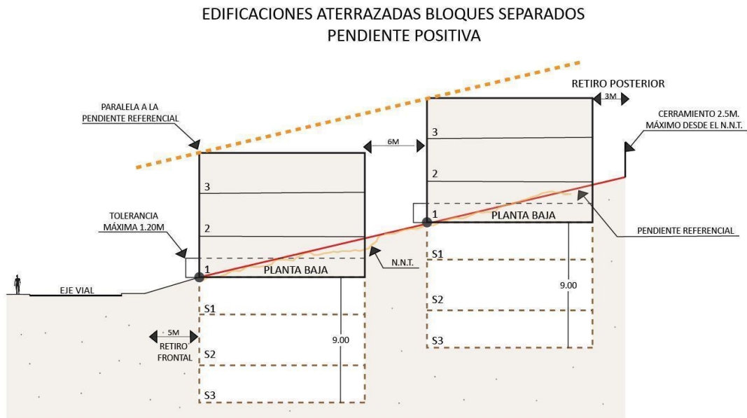
Gráfico 2.026 Edificaciones Aterrazadas Bloques Separados Pendiente Positiva
