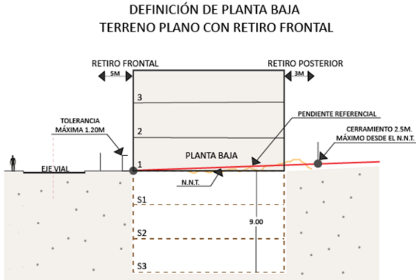
Gráfico 2.017 Definición de Planta Baja en Terreno Plano con Retiro Frontal
