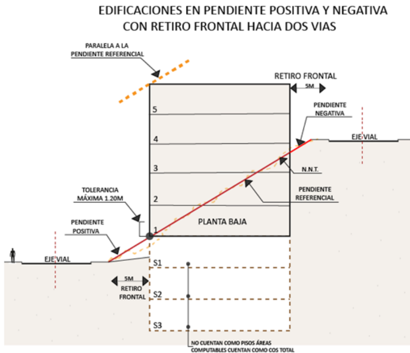
Gráfico 2.018 Edificaciones con Pendiente Positiva o Negativa
