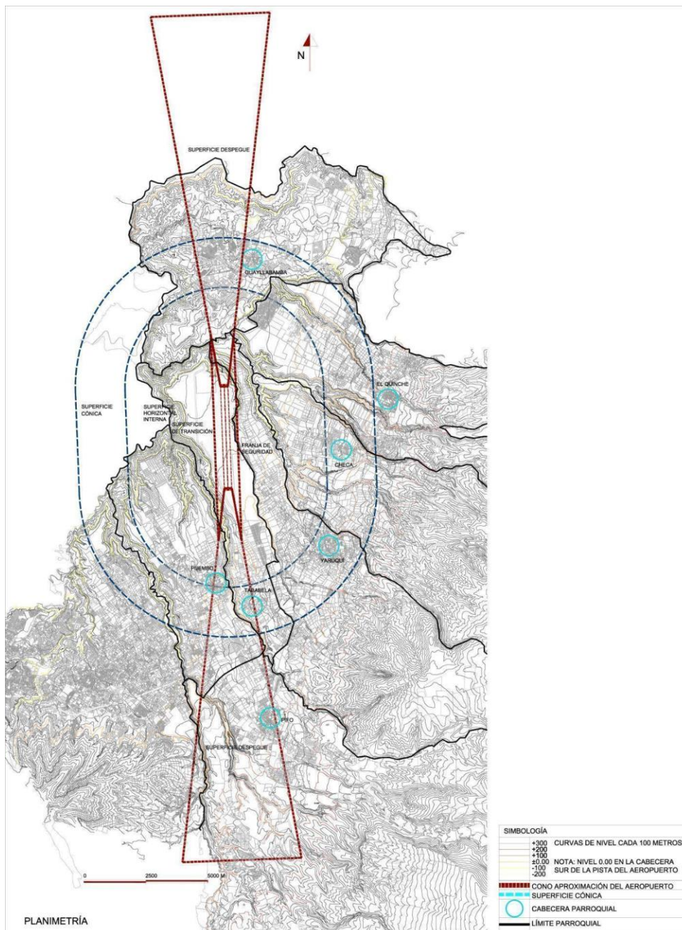
Gráfico 2.042 Superficies limitadoras de obstáculos sobre las parroquias rurales de Puenbo, Pifo, Tababela, Yaruquí, Checa, Guayllabamba y El Quinche.
