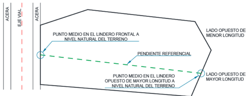
Gráfico 2.014 Pendiente Referencial en Terrenos Irregulares
