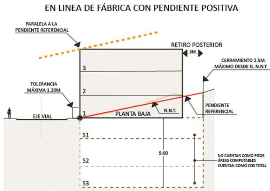
Gráfico 2.019 En Línea de Fábrica con Pendiente Positiva
