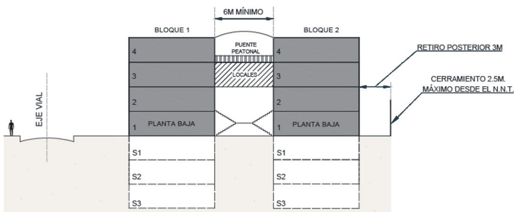
Gráfico 2.032 Edificaciones en Bloques Separados
