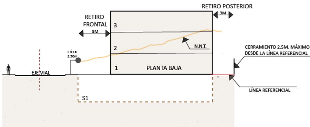
Gráfico 2.027 Edificaciones Aterrazadas en Pendiente Positiva (a)
