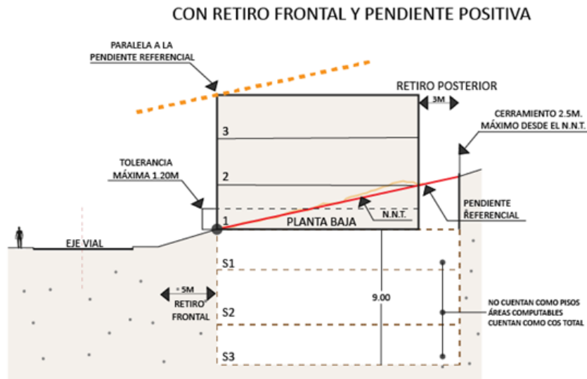
Gráfico 2.020 Con Retiro Frontal y Pendiente Positiva
