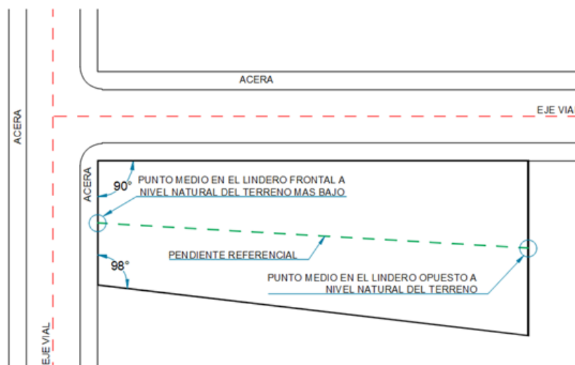
Gráfico 2.013 Pendiente Referencial en Terrenos Esquineros
