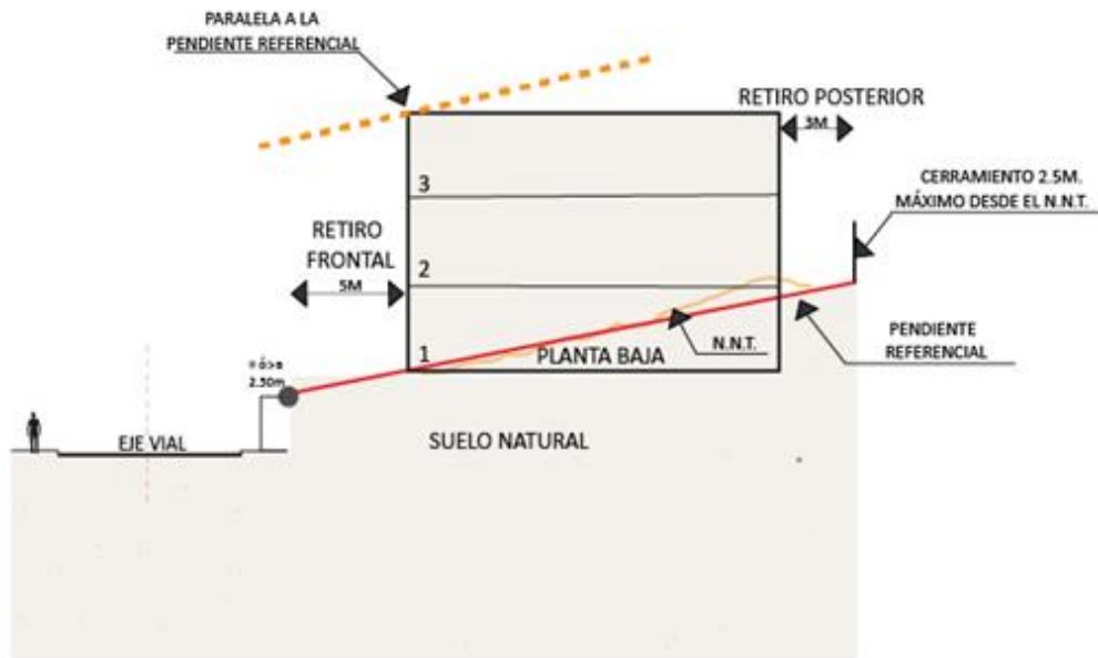
Gráfico 2.028 Edificaciones Aterrazadas en Pendiente Positiva (b)
