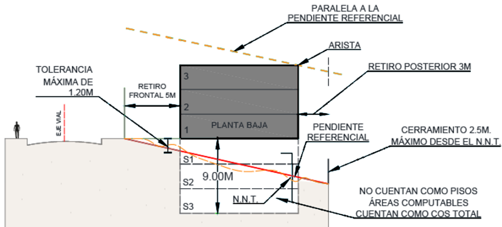
Gráfico 2.022 Con Retiro Frontal y Pendiente Negativa
