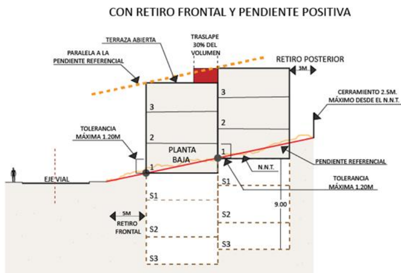
Gráfico 2.023 Retiro Frontal y Pendiente Positiva
