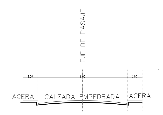
CORTE 1'-1' CALLE CRUZ LOMA ESC. 1/50
