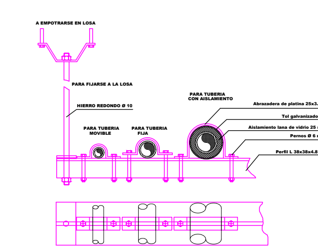
DETALLES CONEXIÓN SISTEMA DE AGUAS SERVIDAS ESC: S/E
