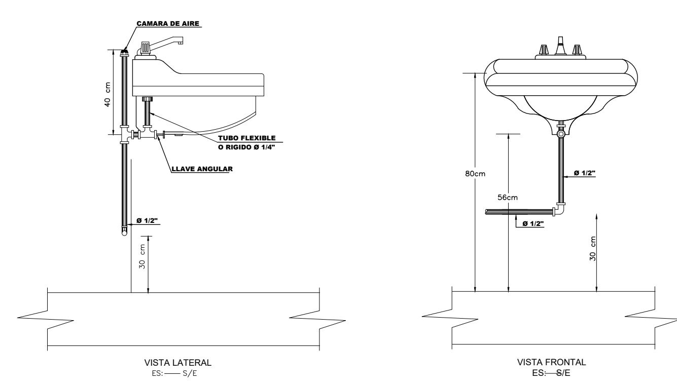
DETALLES CONEXIÓN SISTEMA DE AGUA POTABLE ESC: S/E
