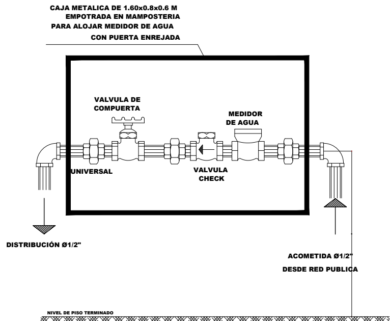
DETALLES CONEXIÓN SISTEMA DE AGUA POTABLE ESC: S/E
