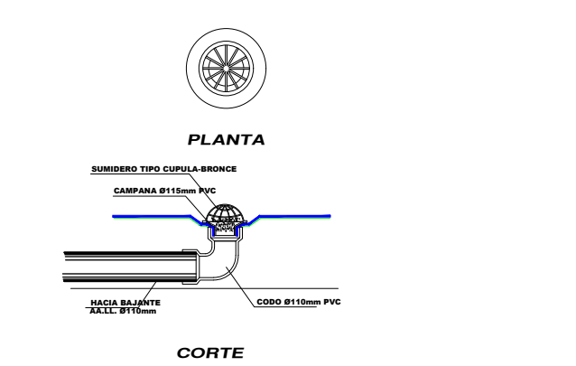
DETALLES SUMIDERO SISTEMA DE AGUAS LLUVIAS ESC: S/E
