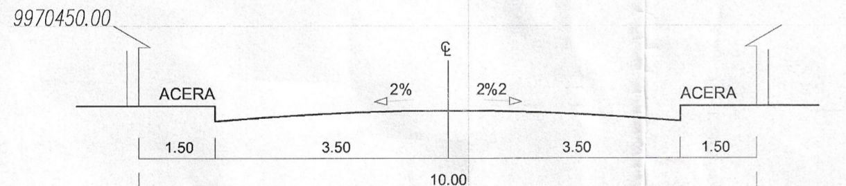
CALLE AURELIO ESPINOZA POLIT ESCALA: S/E
