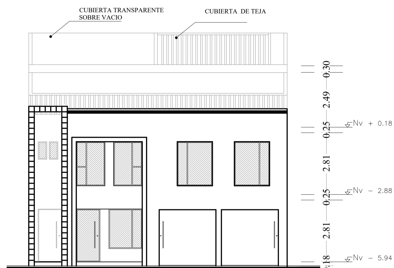
CALLE ANTONIO DE RIVERA FACHADA FRONTAL ESCALA 1:100
