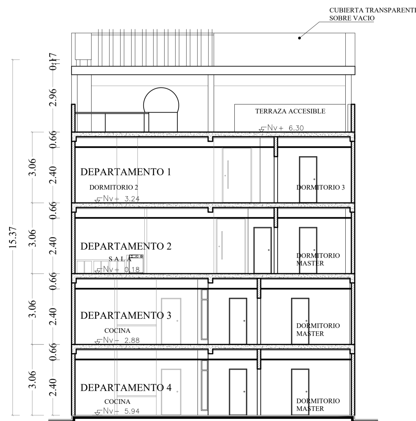
CORTE B - B' ESCALA 1:100
