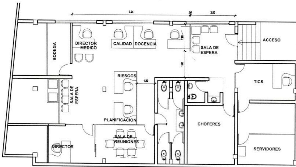
PROPUESTA ADMINISTRACION 2DA PLANTA BLOQUE DE MANTENIMIENTO ESCALA 1 A 100
