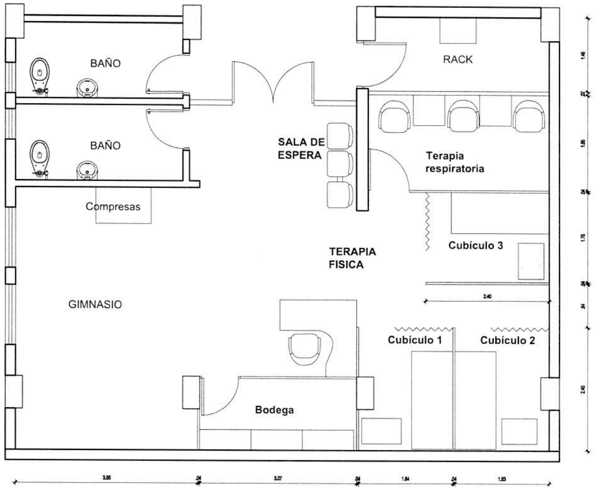
PROPUESTA FISIOTERAPIA PLANTA BAJA BLOQUE 4 ESCALA 1 A 50
