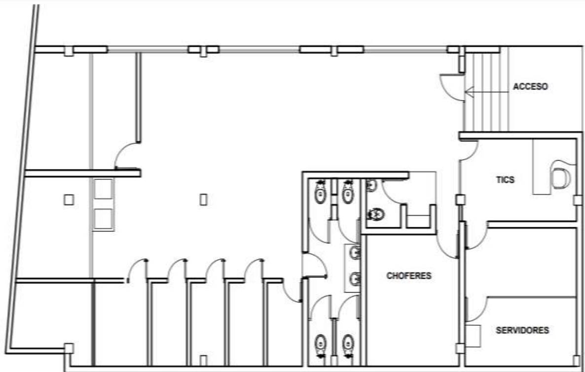
ESTADO ACTUAL - SEGUNDA PLANTA BLOQUE DE MANTENIMIENTO ESCALA 1 A 100
