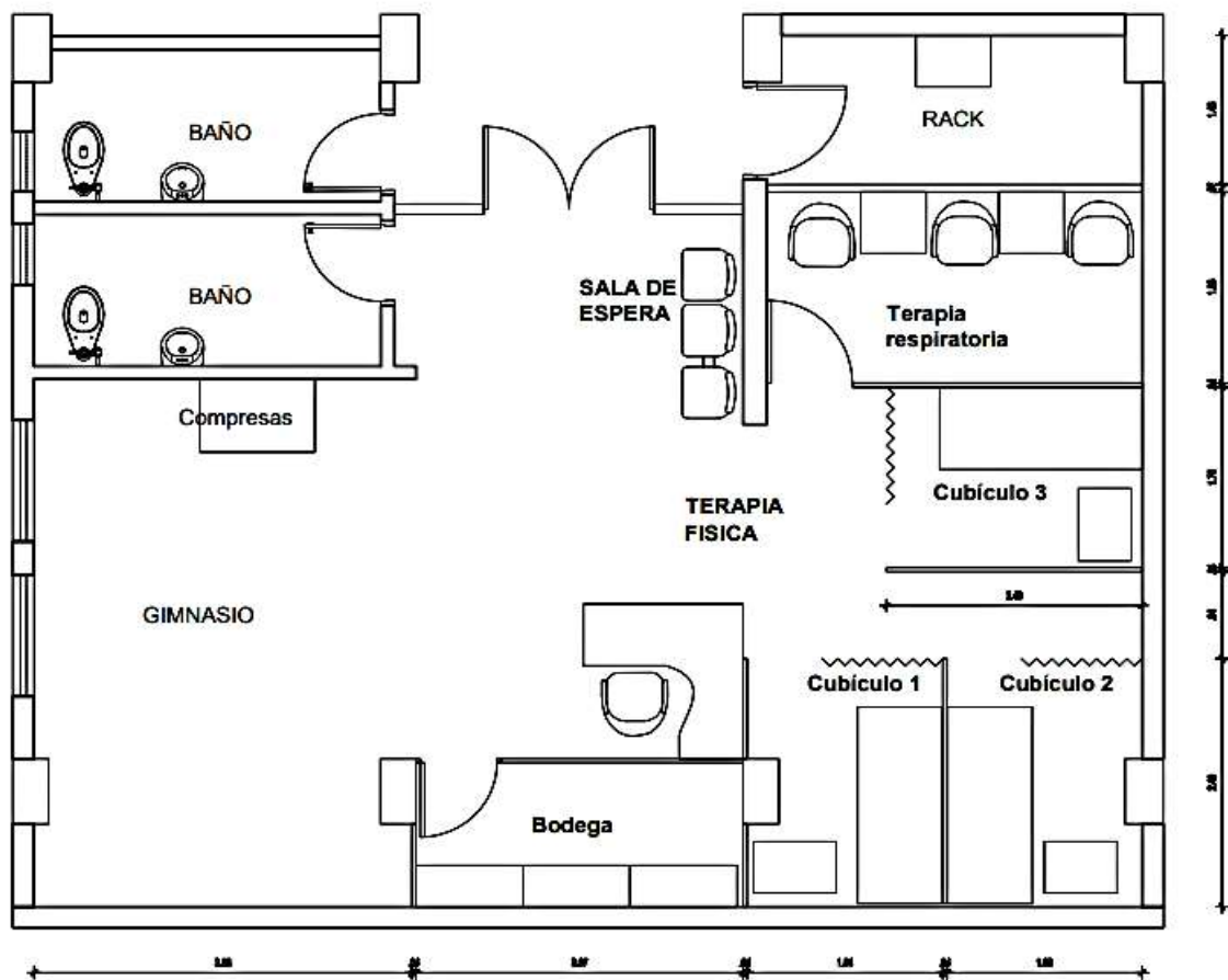
PROPUESTA FISIOTERAPIA PLANTA BAJA BLOQUE 4 ESCALA 1 A 50
