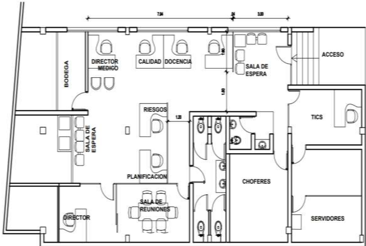
PROPUESTA ADMINISTRACION 2DA PLANTA BLOQUE DE MANTENIMIENTO ESCALA 1 A 100
