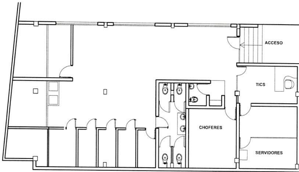
ESTADO ACTUAL - SEGUNDA PLANTA BLOQUE DE MANTENIMIENTO ESCALA 1 A 100
