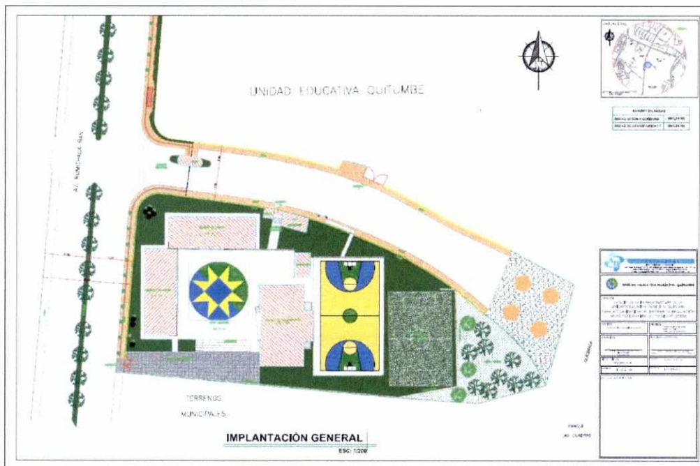
Gráfico No. 4 Implantación general del ex Colegio Municipal Gral. Luis Telmo Paz y Miño hoy parte de la Unidad Educativa Municipal "Quitumbe".
