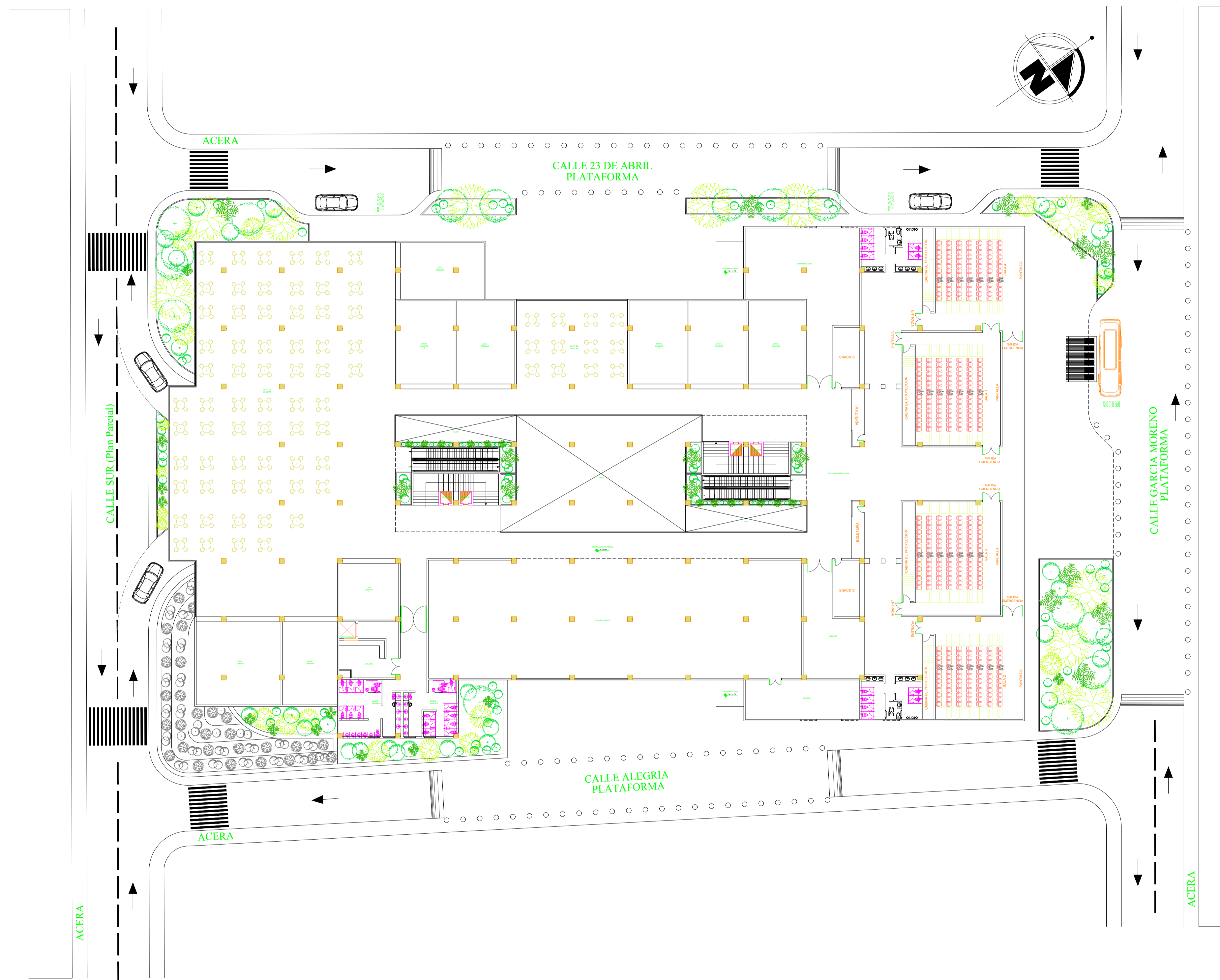
TERCERA PLANTA ALTA N+12.60 ESC: 1:100
