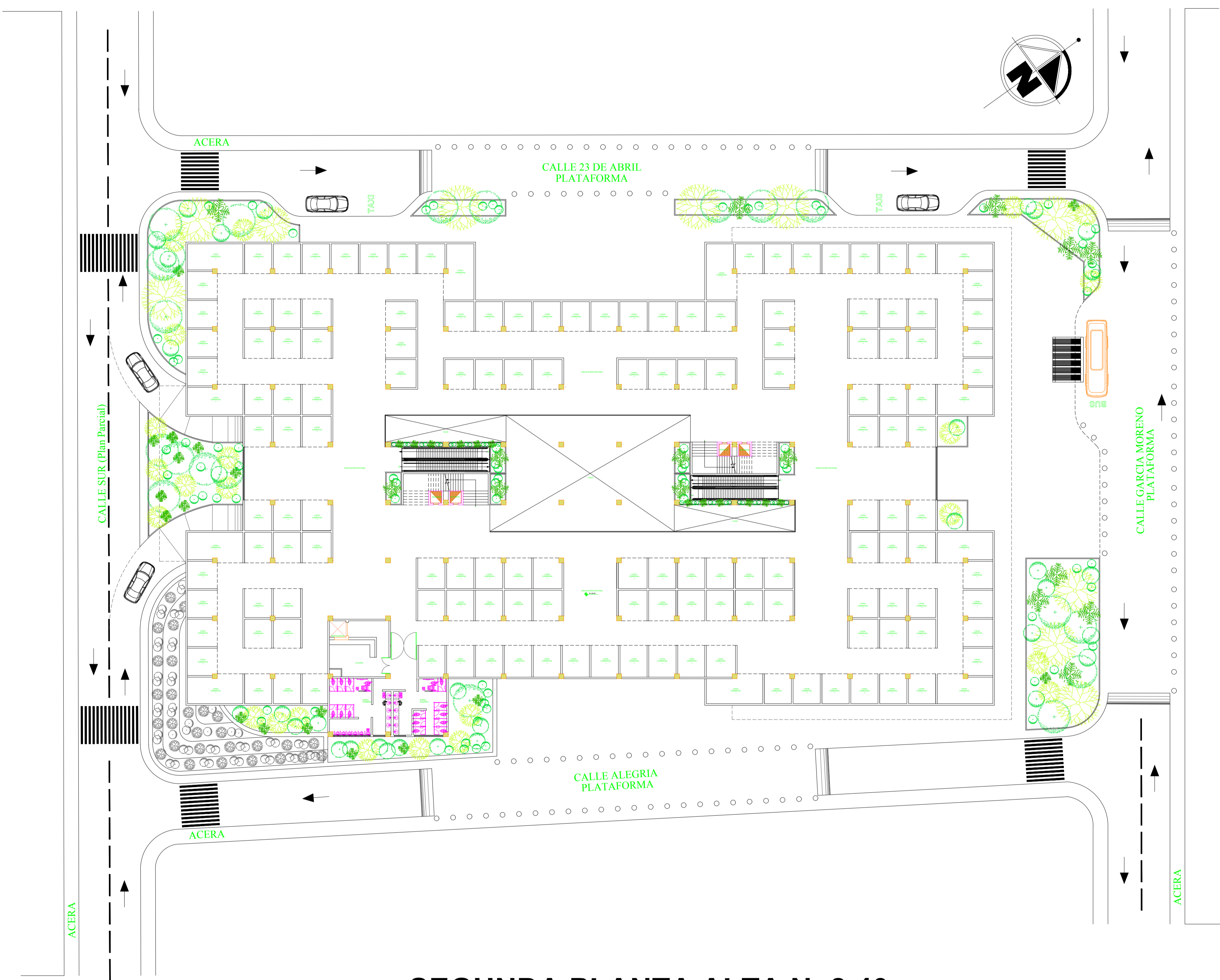
SEGUNDA PLANTA ALTA N+8.40 ESC: 1:100
