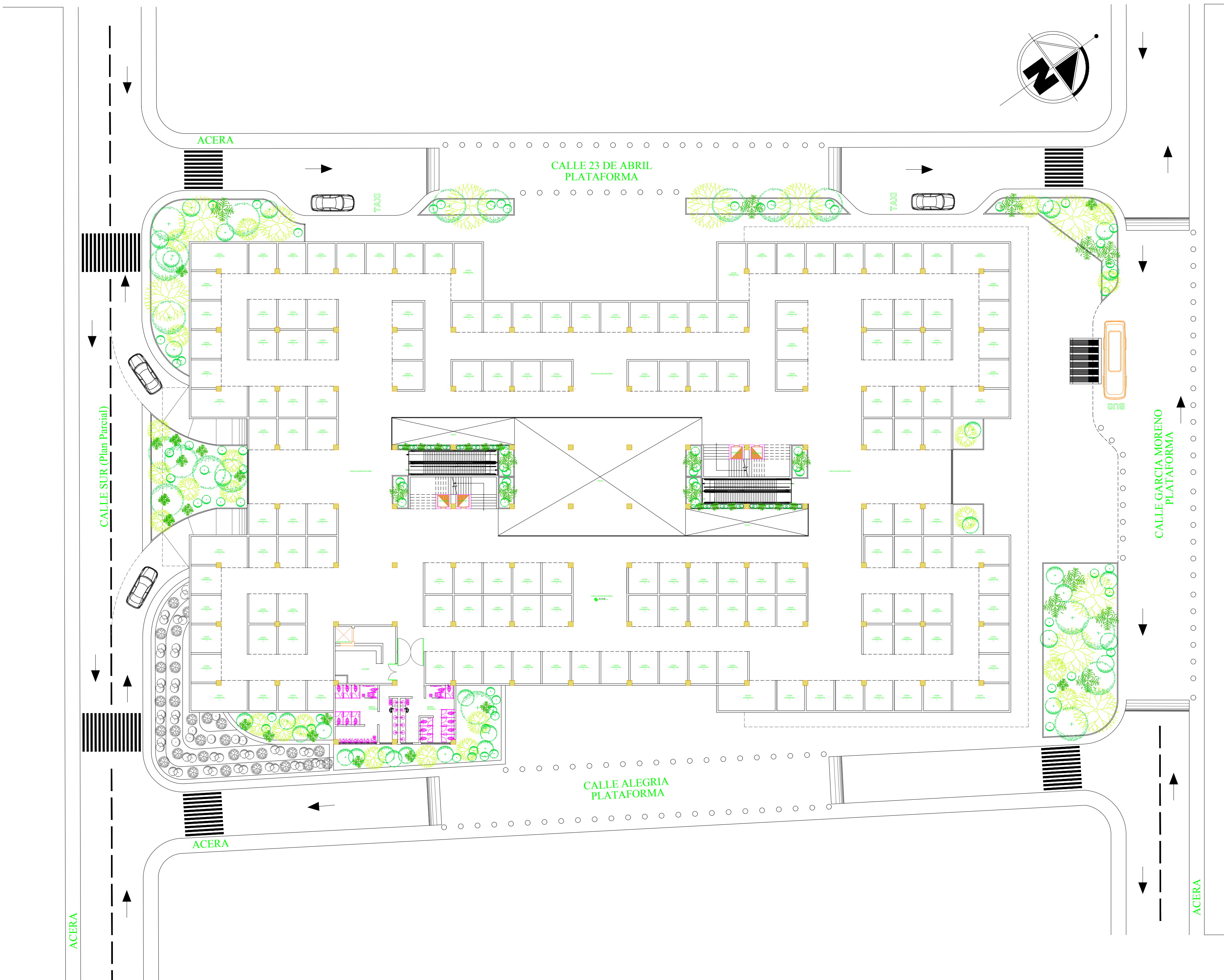
PRIMERA PLANTA ALTA N+4.20 ESC: 1:100
