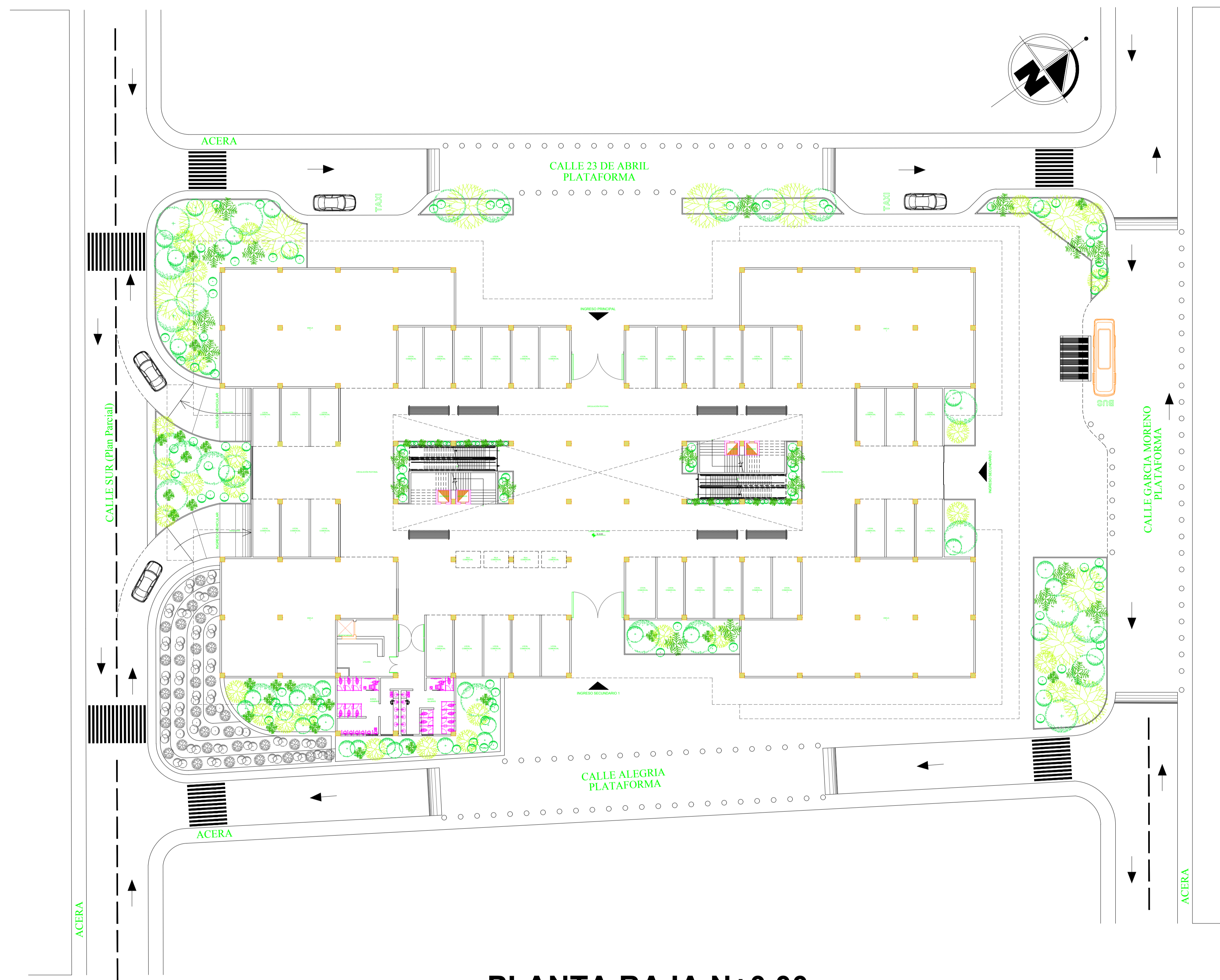
PLANTA BAJA N+0.00 ESC: 1:100
