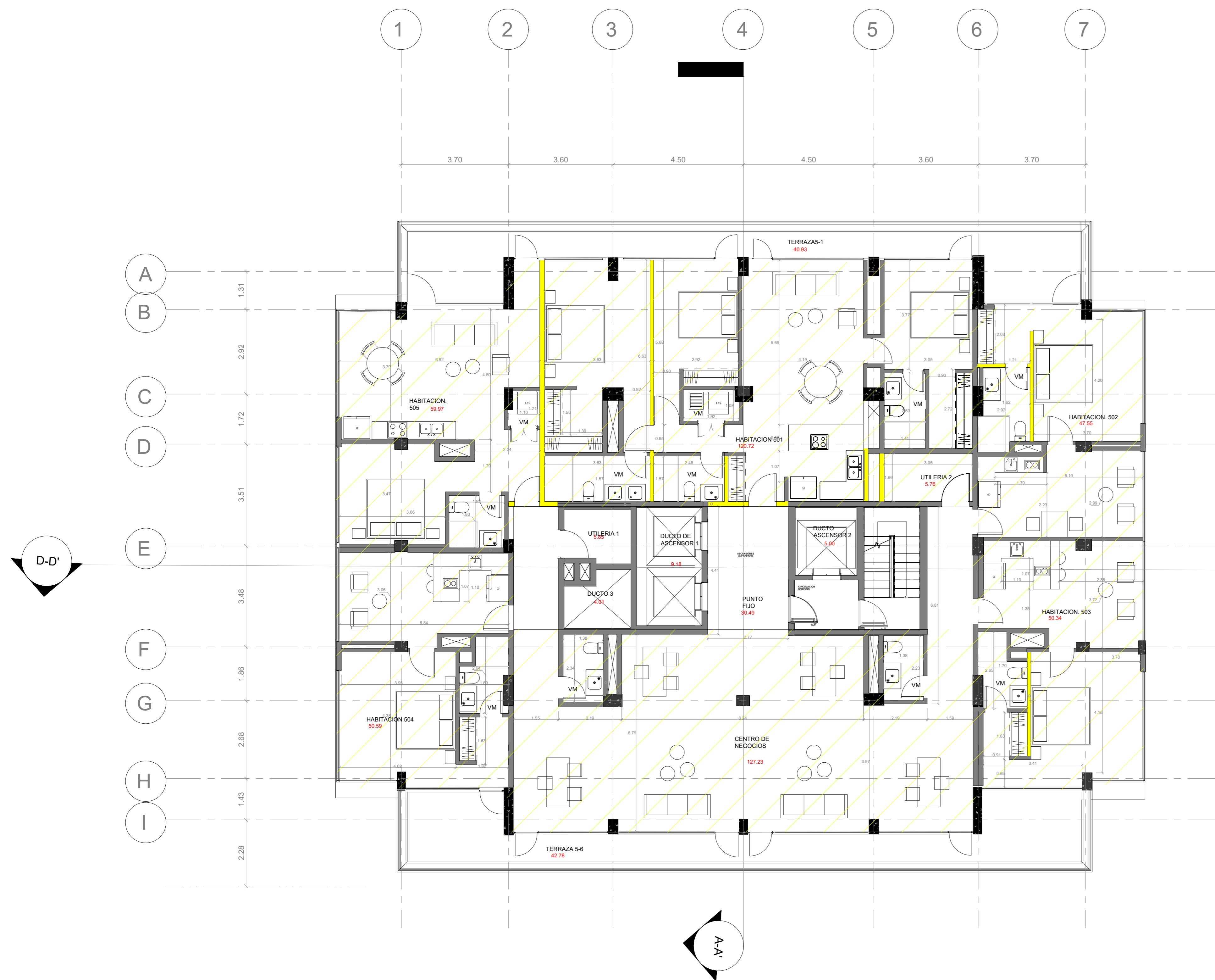
1 PISO 5 1 : 75 Nivel: +12.00
