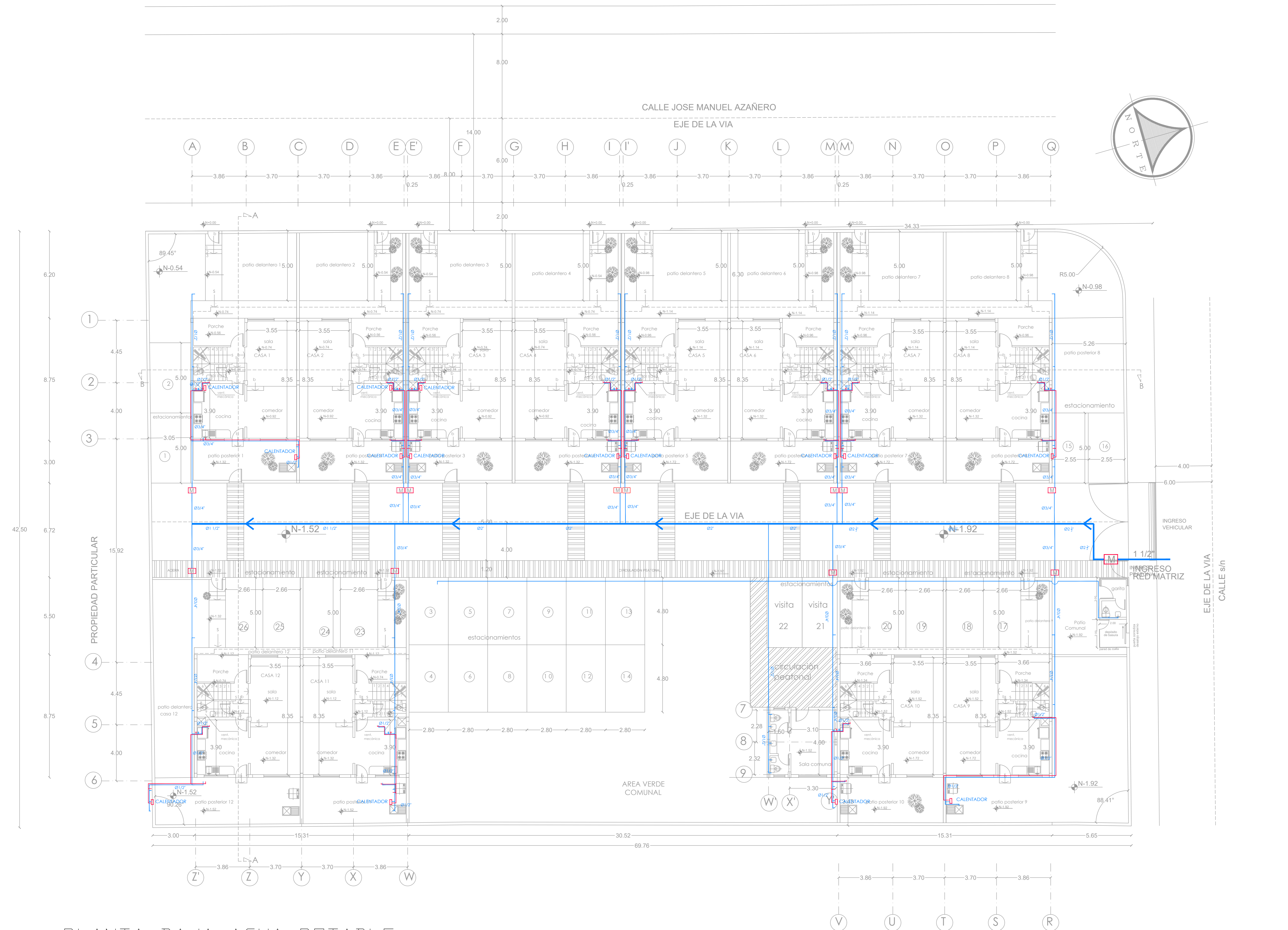
PLANTA BAJA AGUA POTABLE ESCALA 1=100
