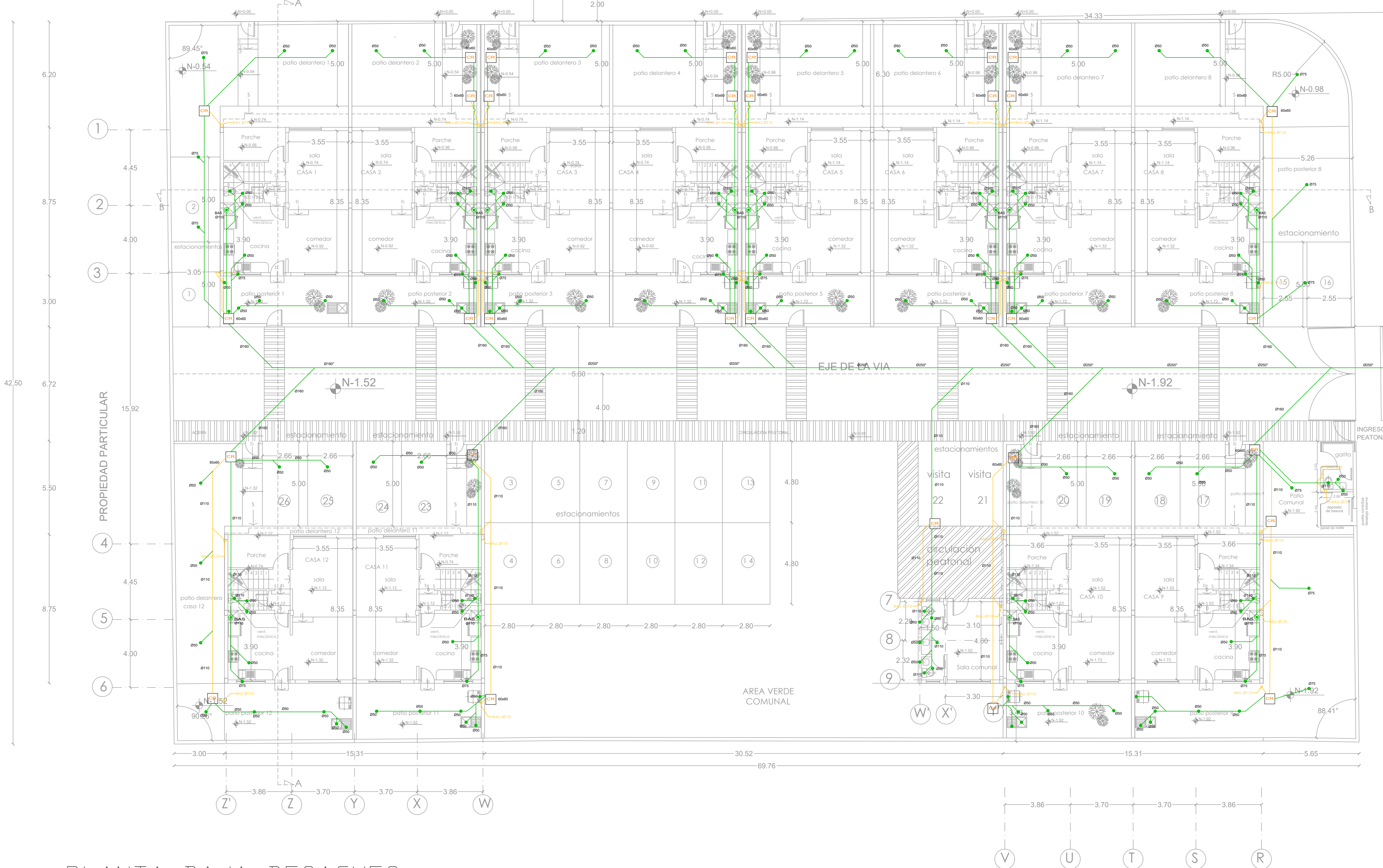
PLANTA BAJA DESAGUES ESCALA 1=100
