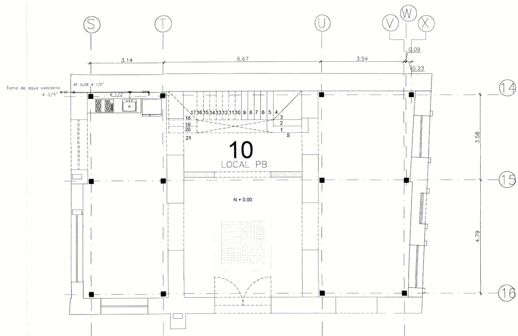
Planta Baja Escala ----- 1:100
