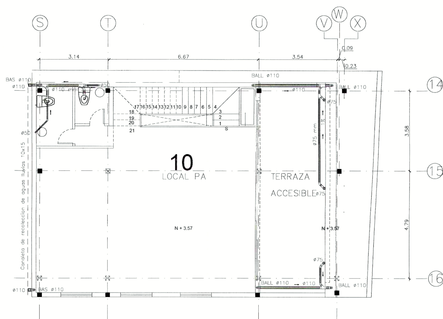
Planta Alta Escala ----- 1:100
