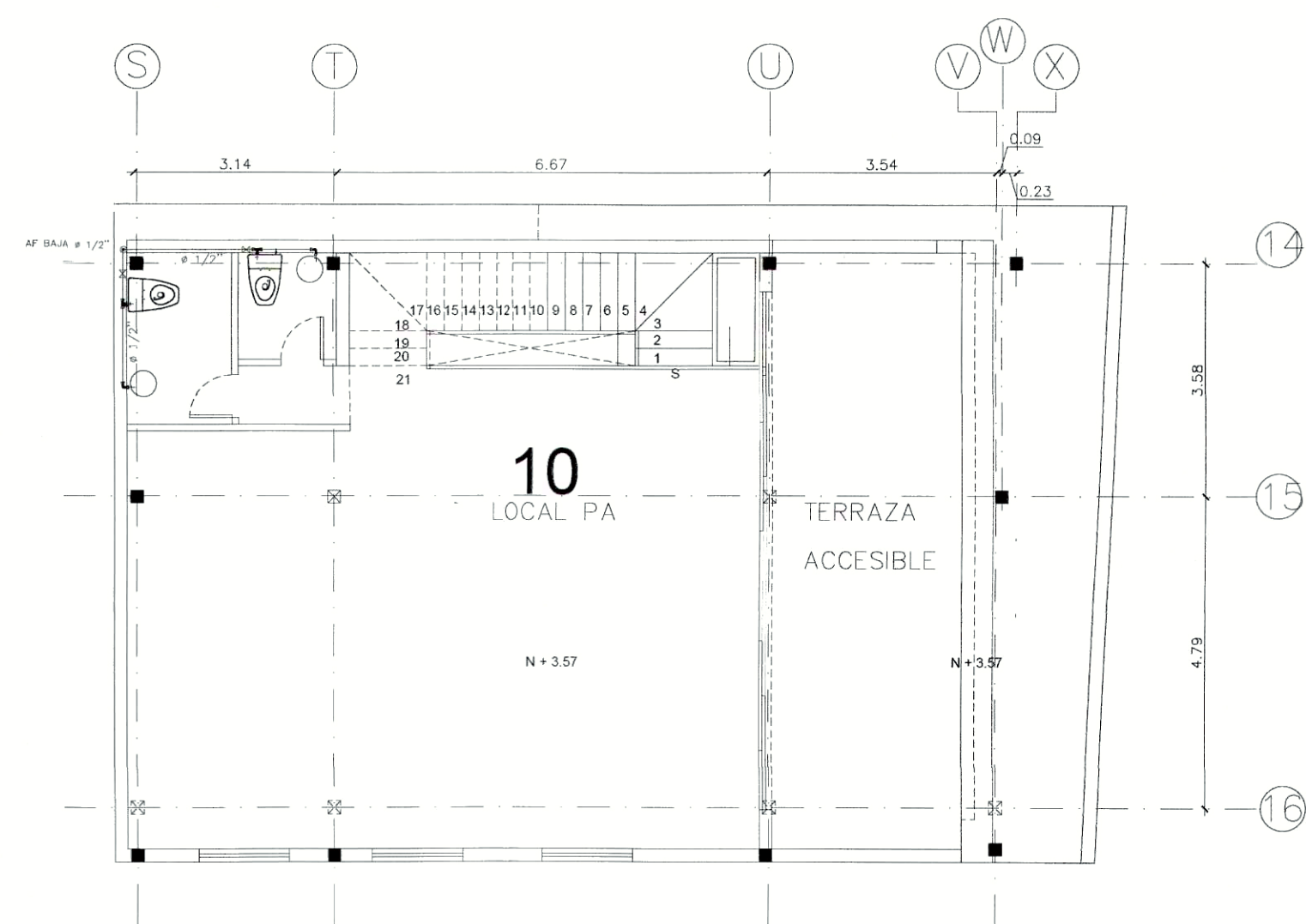
Planta Alta Escala ----- 1:100
