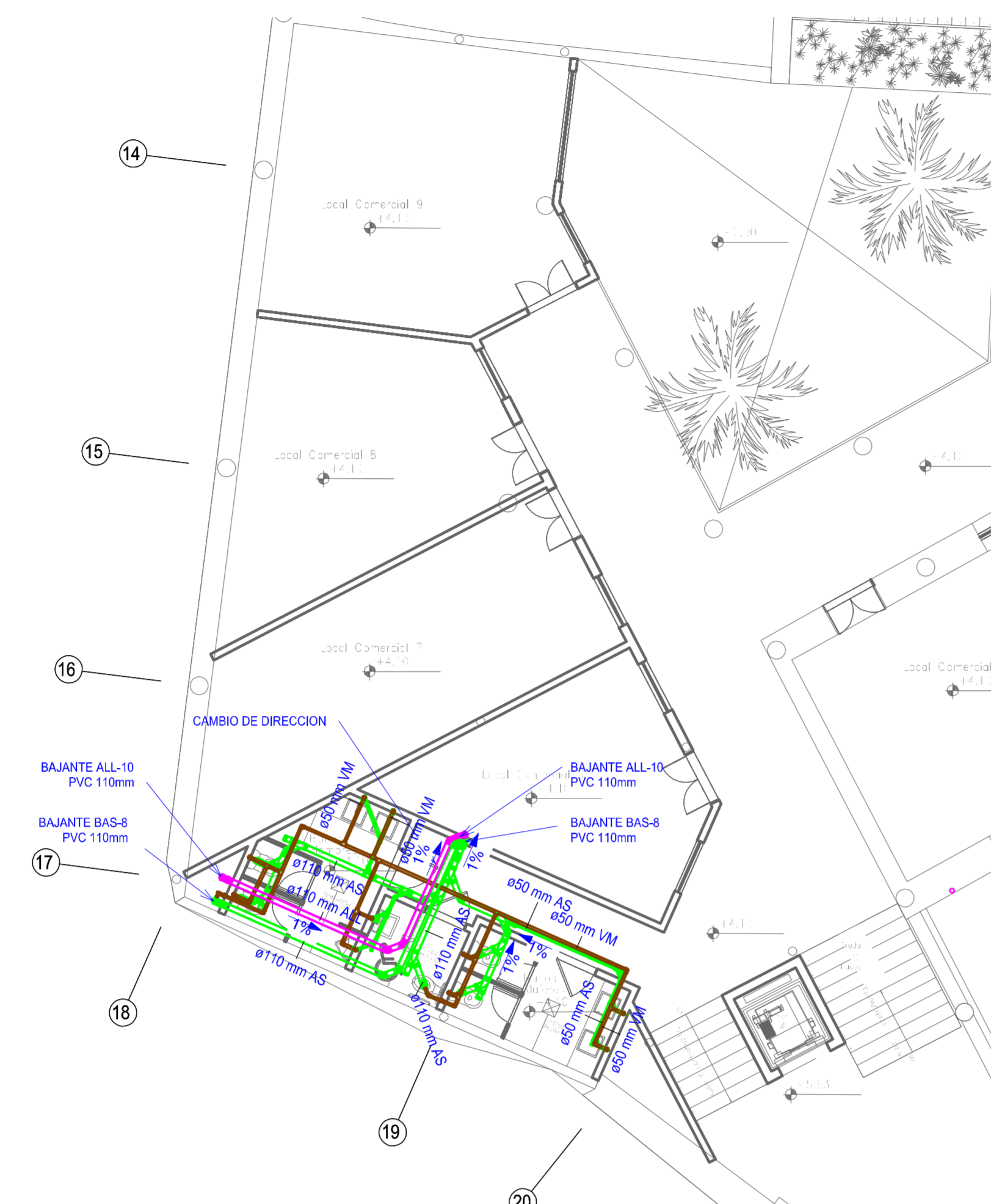
1 3.1 NIVEL +4.10 -SECTOR A ESC: 1:100
