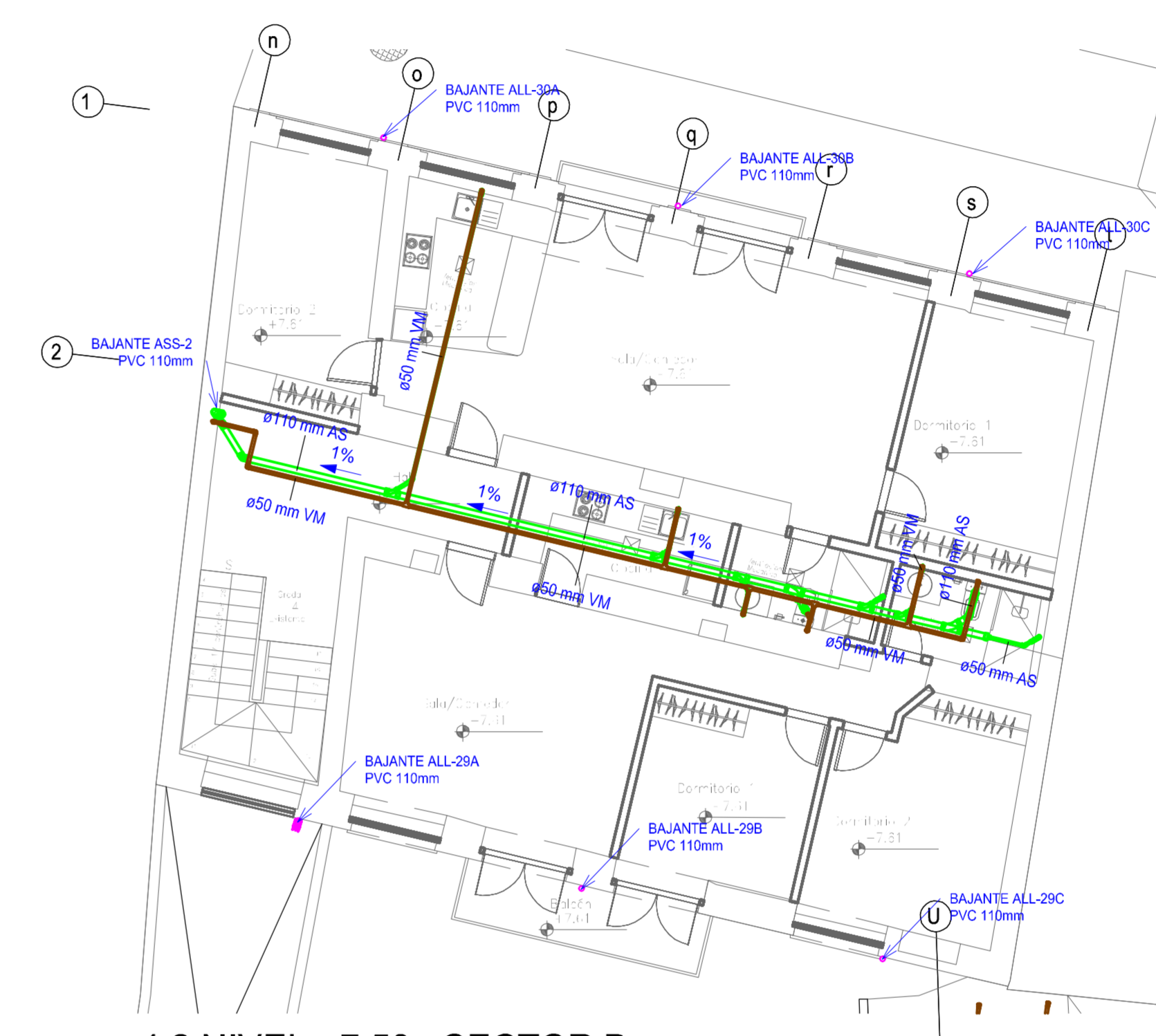
2 4.2 NIVEL +7.50 - SECTOR B ESC: 1:100
