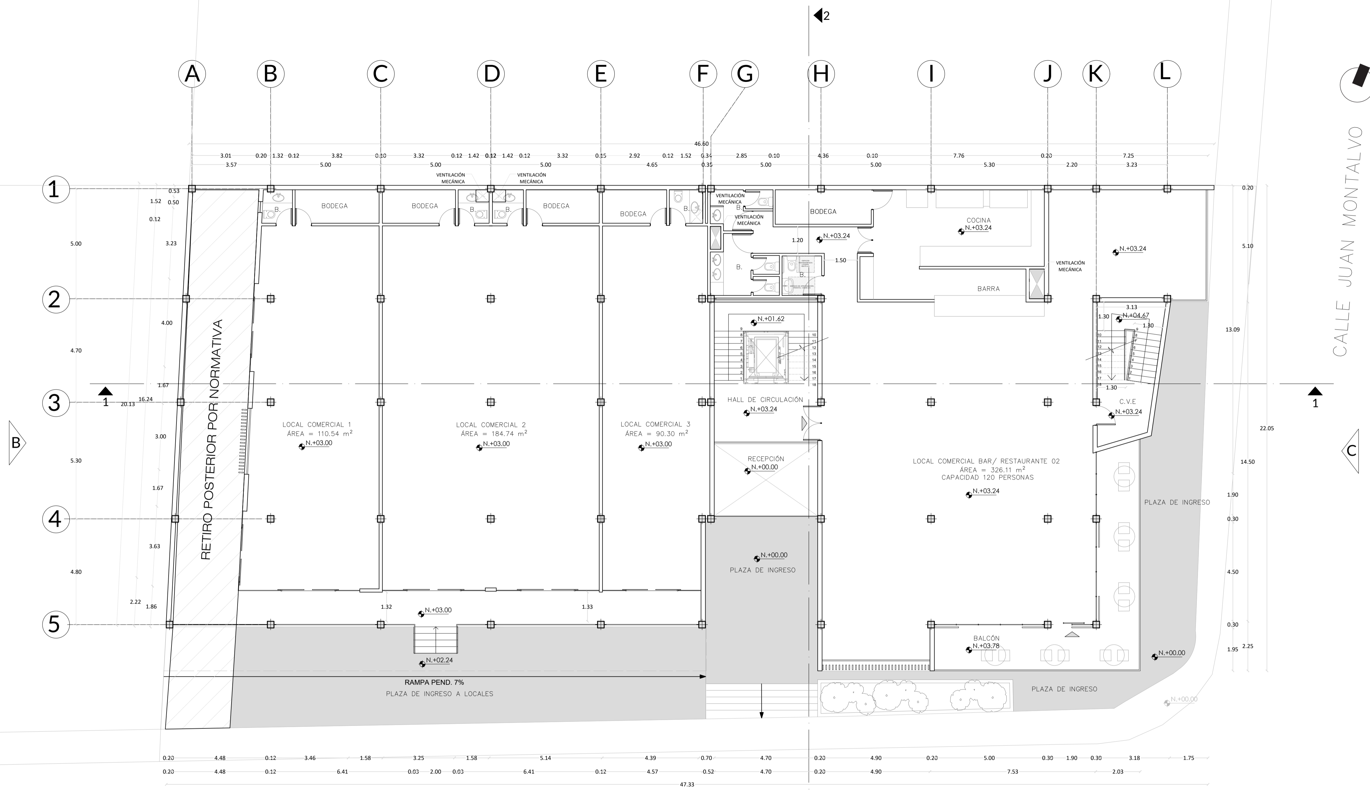
PLANTA ARQUITECTÓNICA NIVEL (+3.24) ESC.: 1:100
