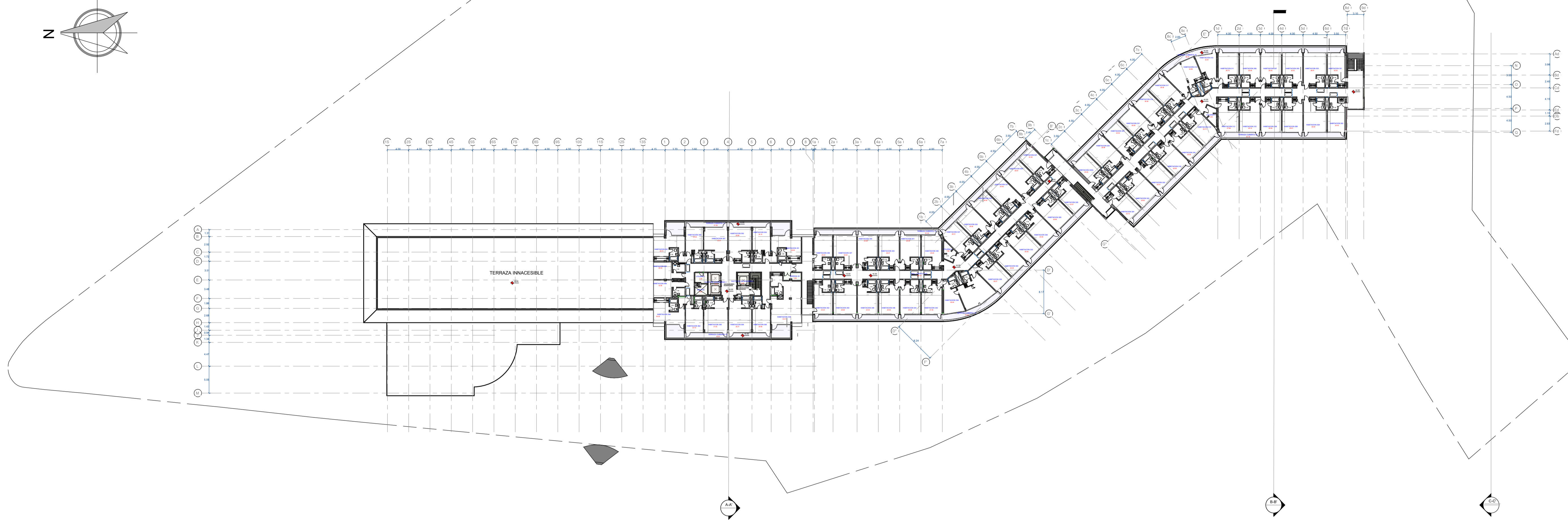
1 PISO 3 1 : 250
