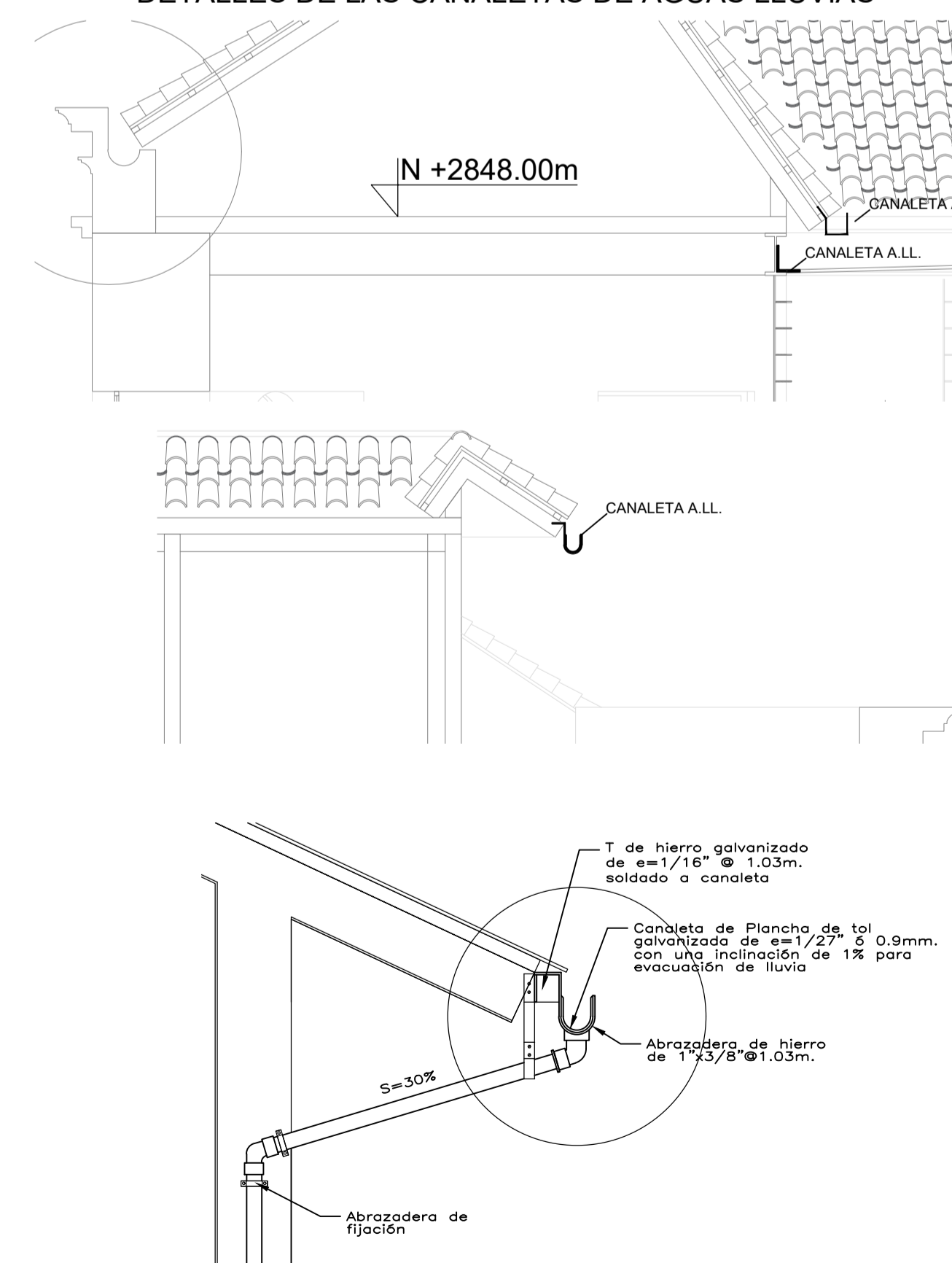
DETALLES DE LAS CANALETAS DE AGUAS LLUVIAS
