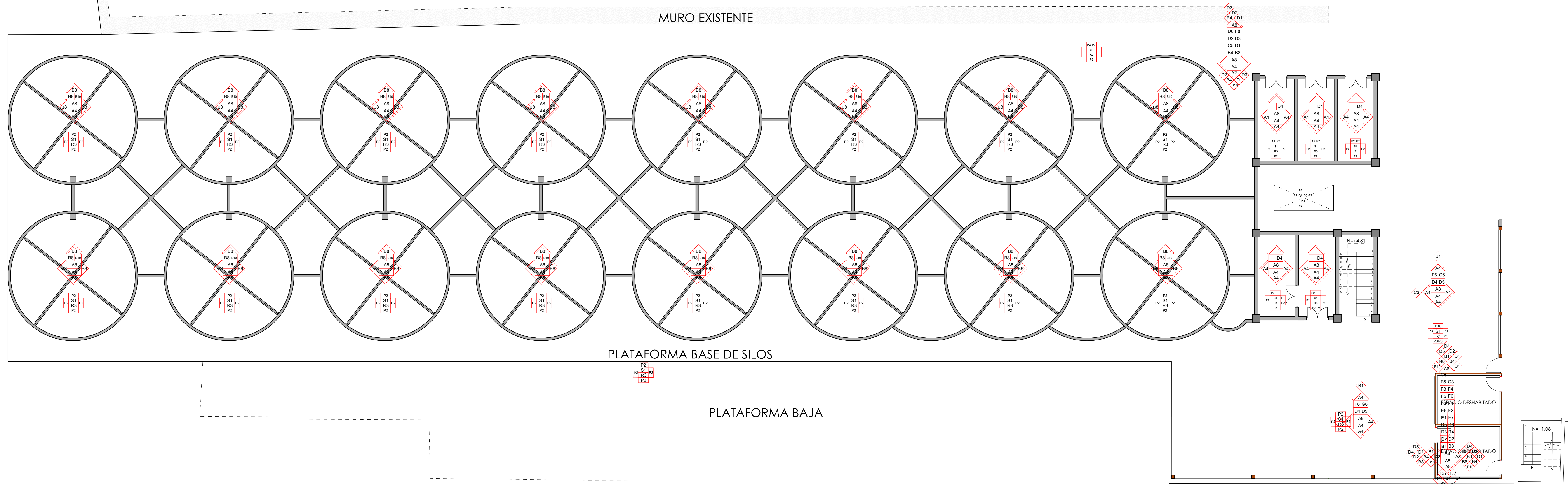
Planta de Silos y casa de maquinas N=+2.04 esc 1:100
