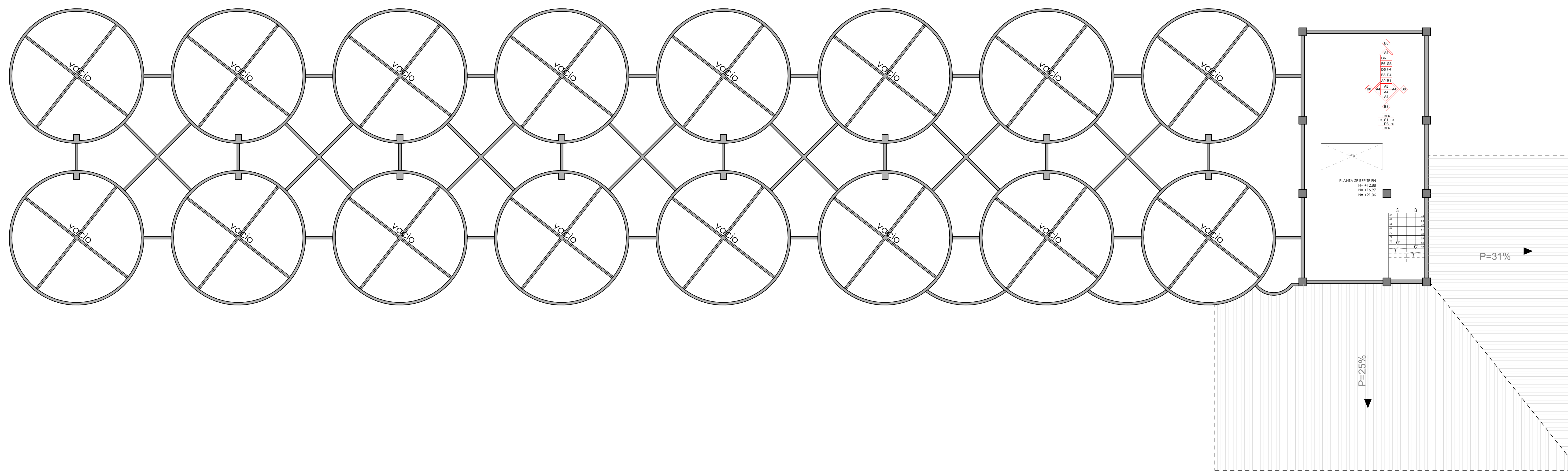
Plantas de Silos y casa de maquinas N=+12.88/+16.97/+21.06 esc 1:100
