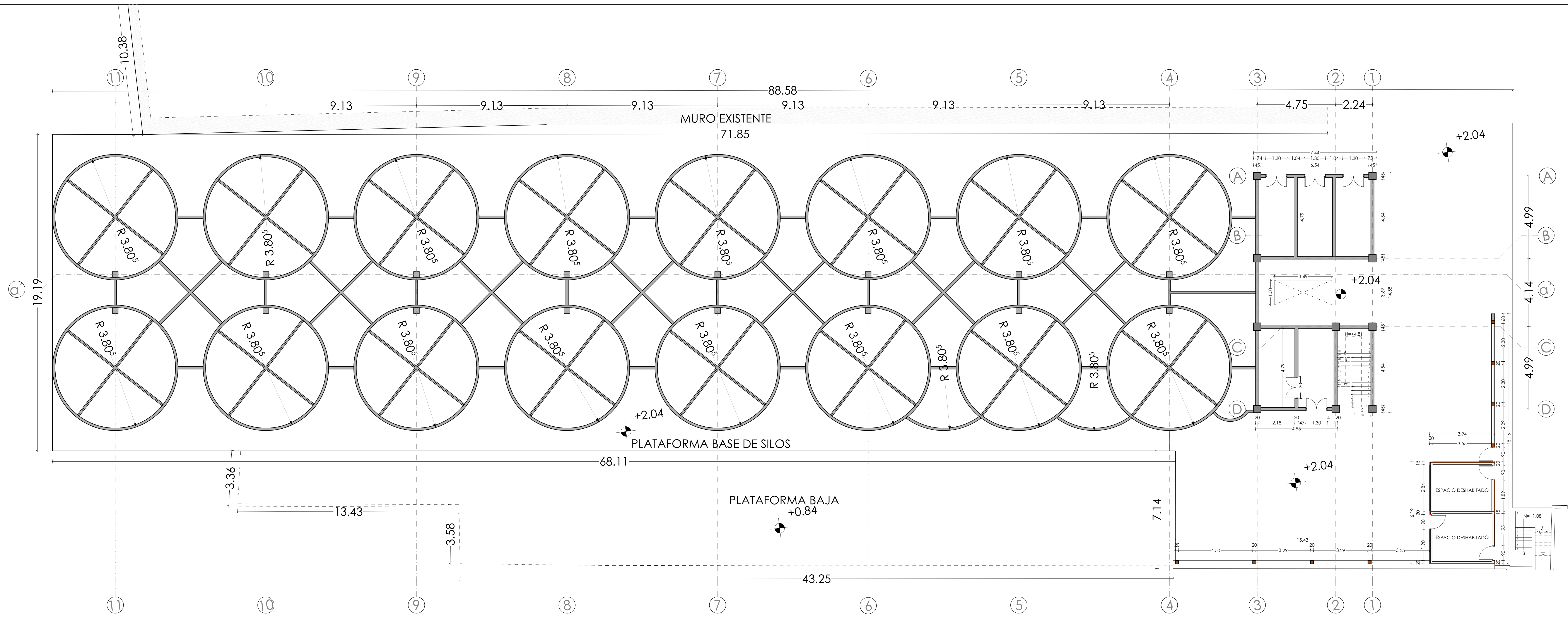
Planta baja de Silos y casa de maquinas N=+2.04 esc 1:100
