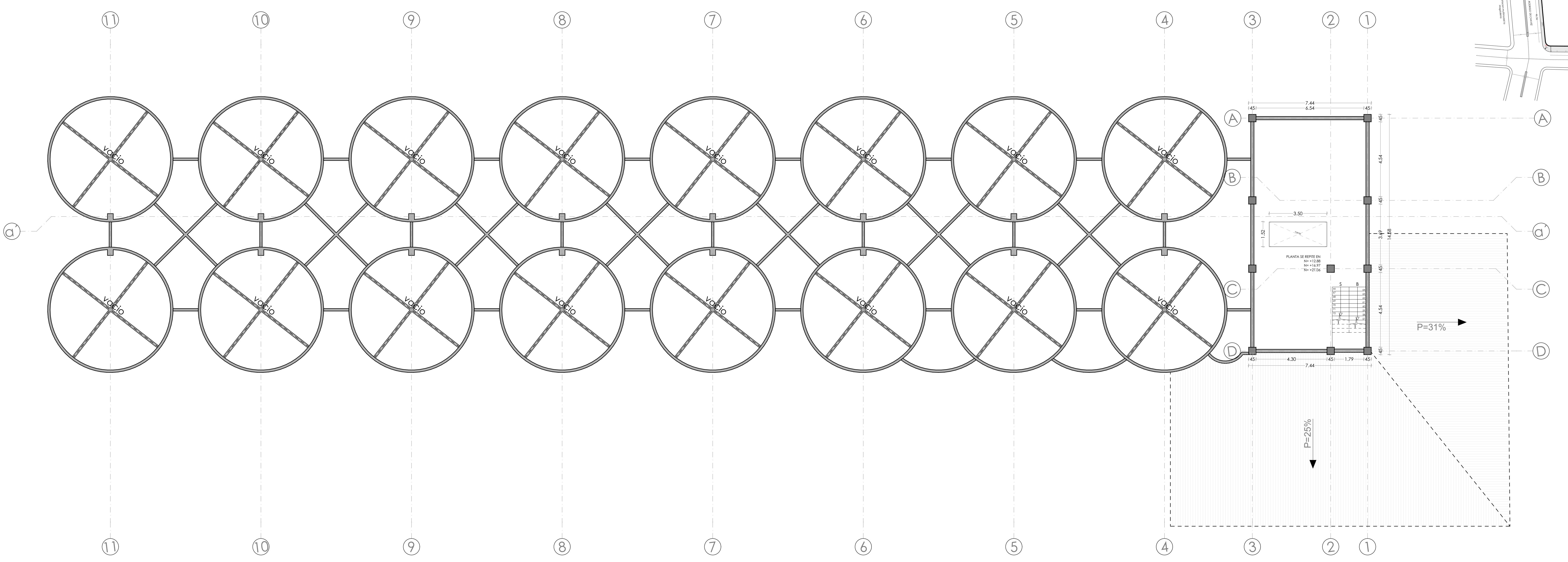
Plantas altas de Silos s N=+12.88/+16.97/+21.06 esc 1:100
