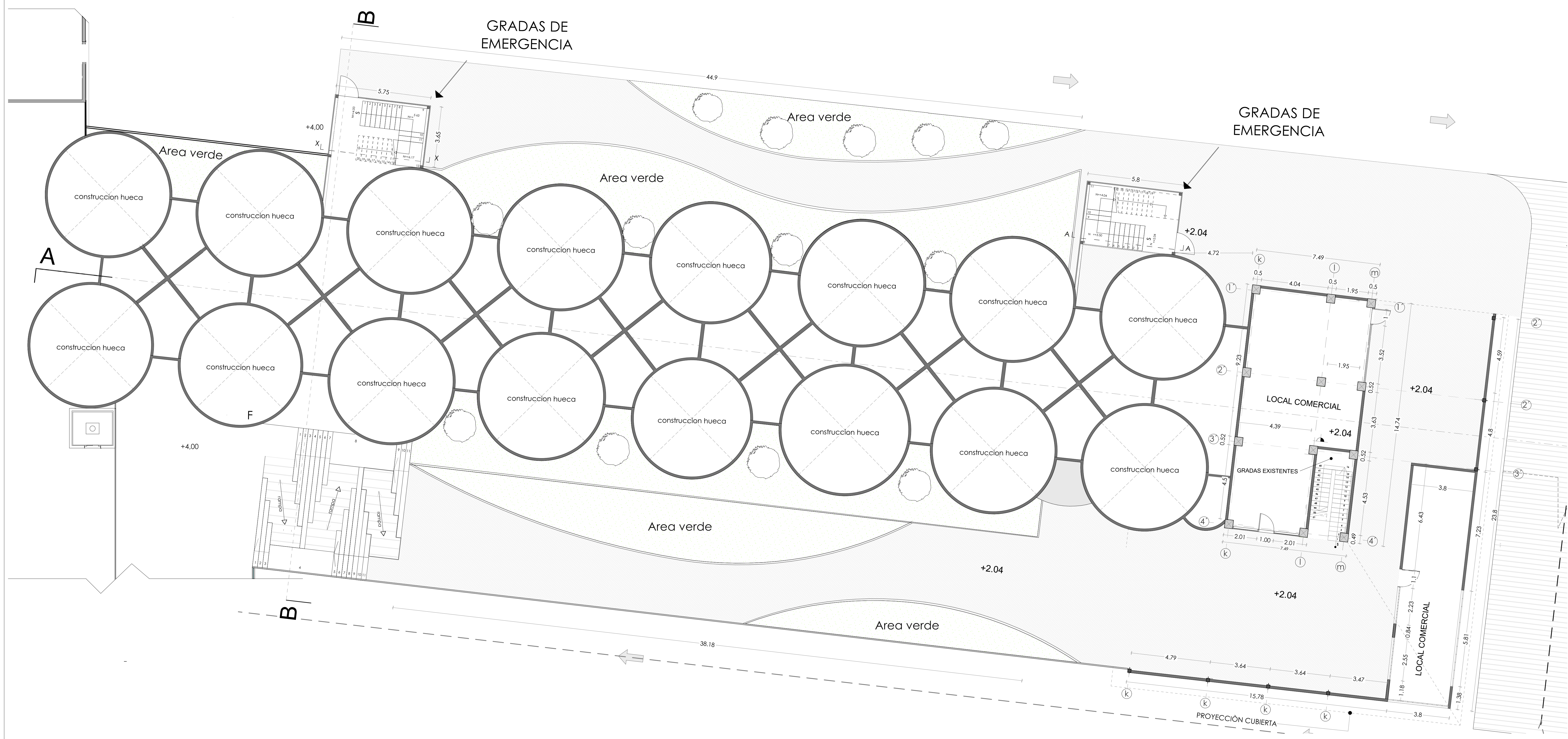
Planta baja base silos N=+2.04 esc 1:100
