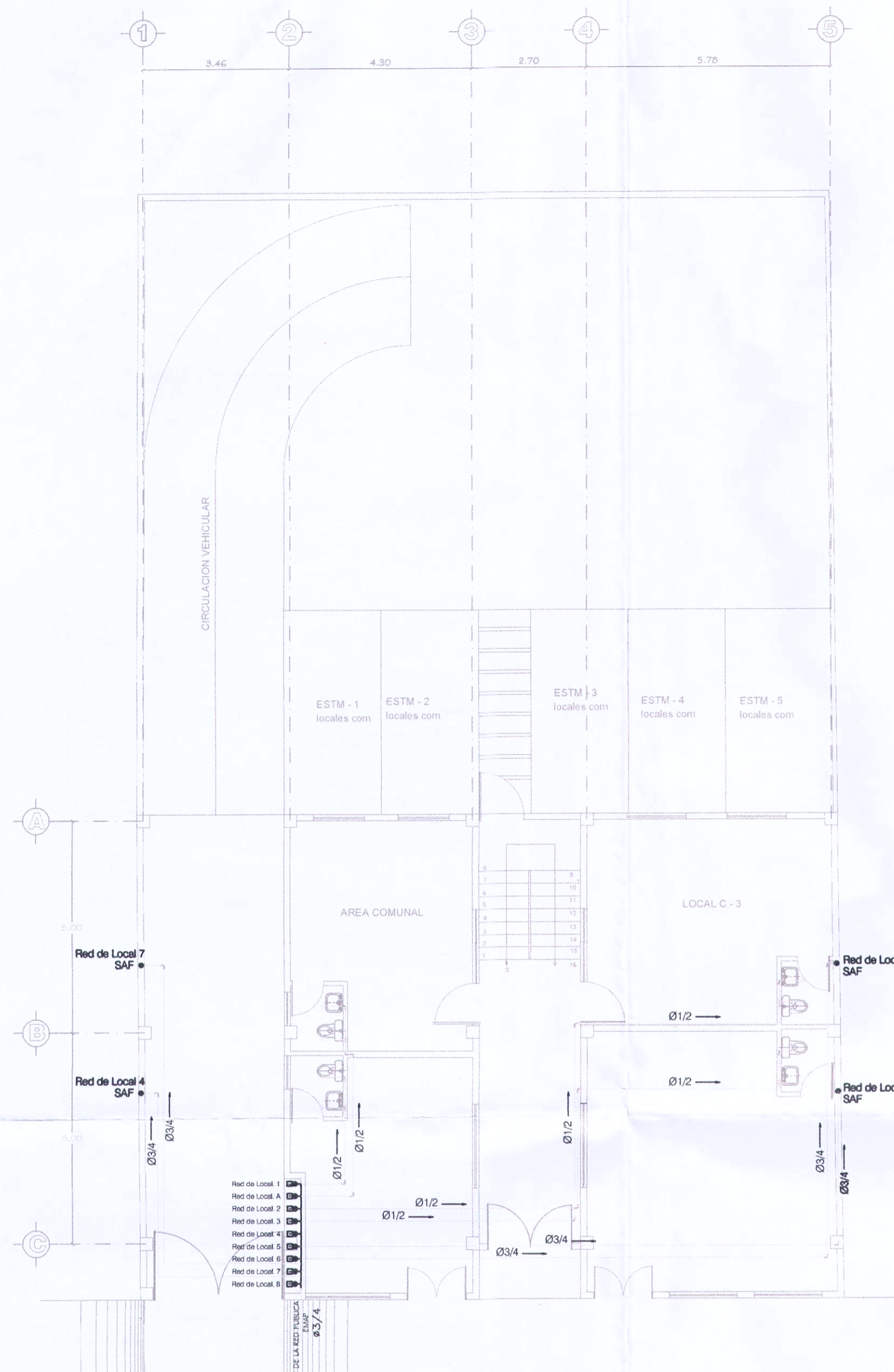
PLANTA BAJA N. + 0.33 ESCALA: 1 : 100
