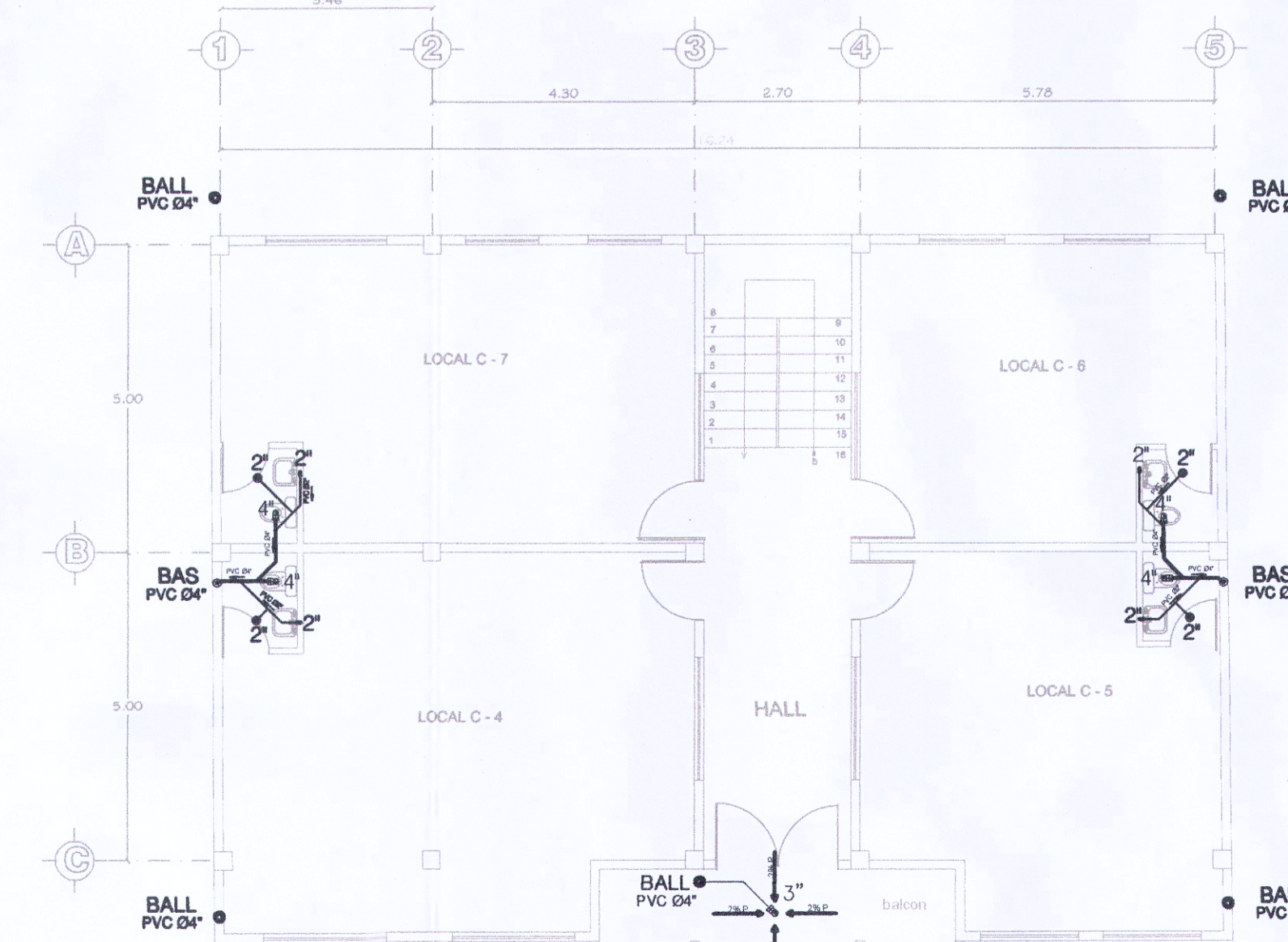
PRIMER PLANTA ALTA N. + 3.05 ESCALA: 1 : 100
