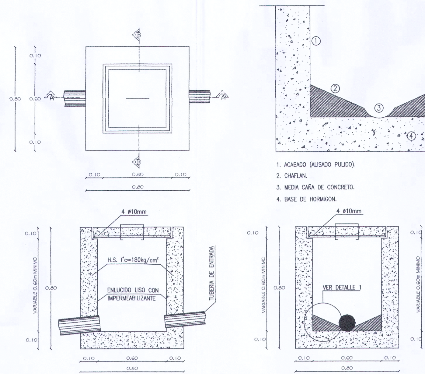
DETALLE DE CAJA DE REVISIÓN SIN ESCALA
