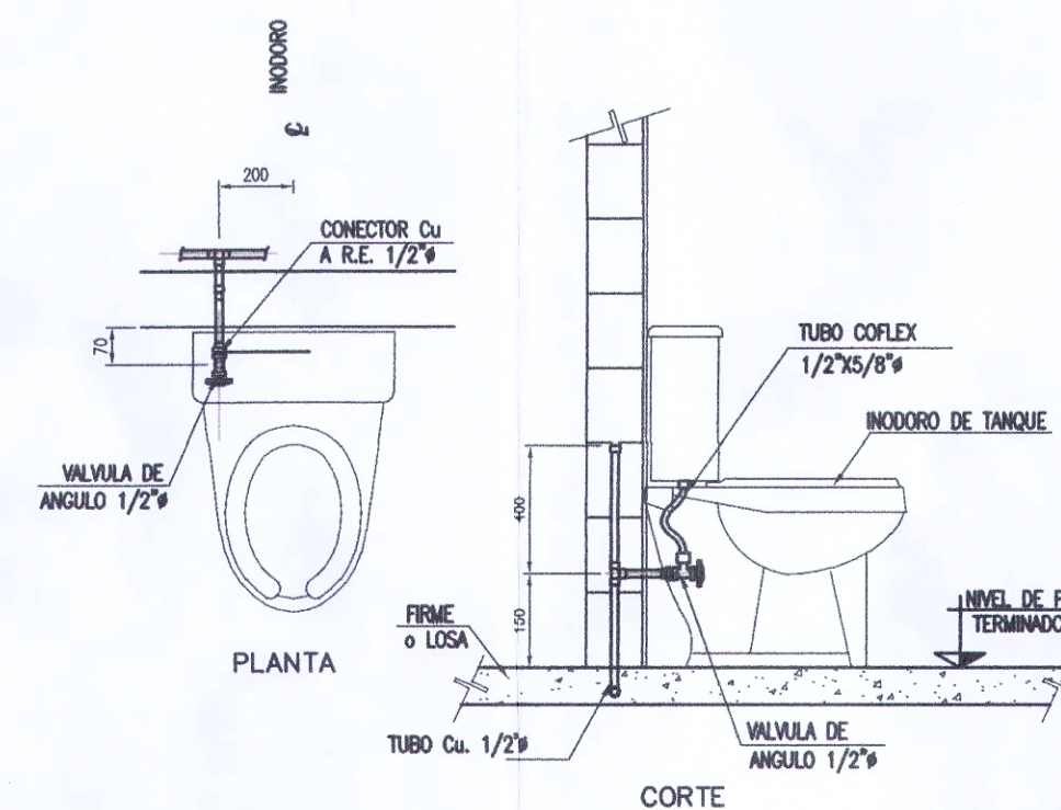
DETALLE DE INODORO SIN ESCALA
