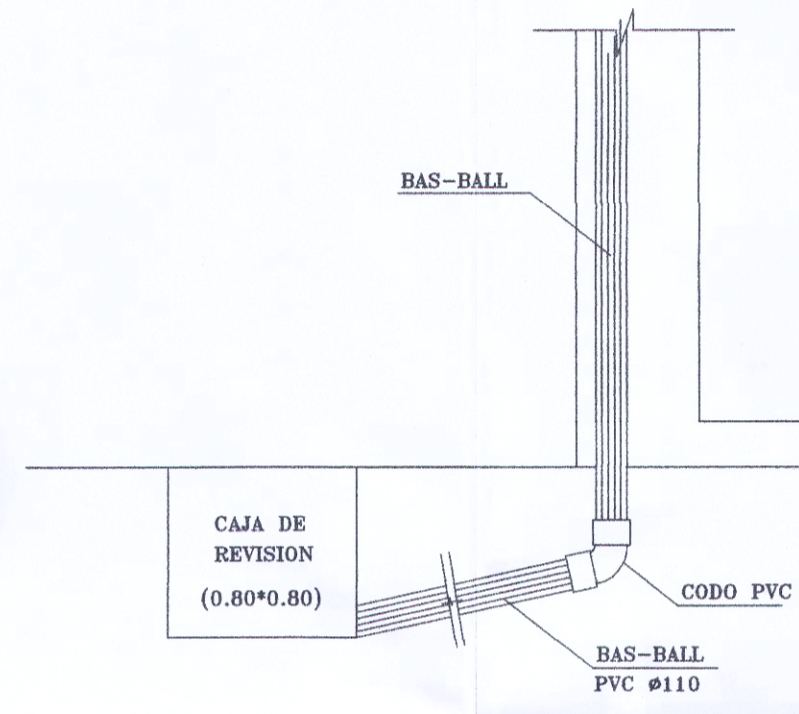
CONEXIÓN BAS-BALL-CAJA DE REVISIÓN SIN ESCALA
