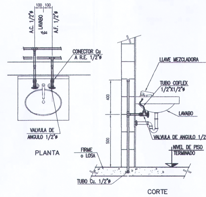
DETALLE DE LAVABO SIN ESCALA
