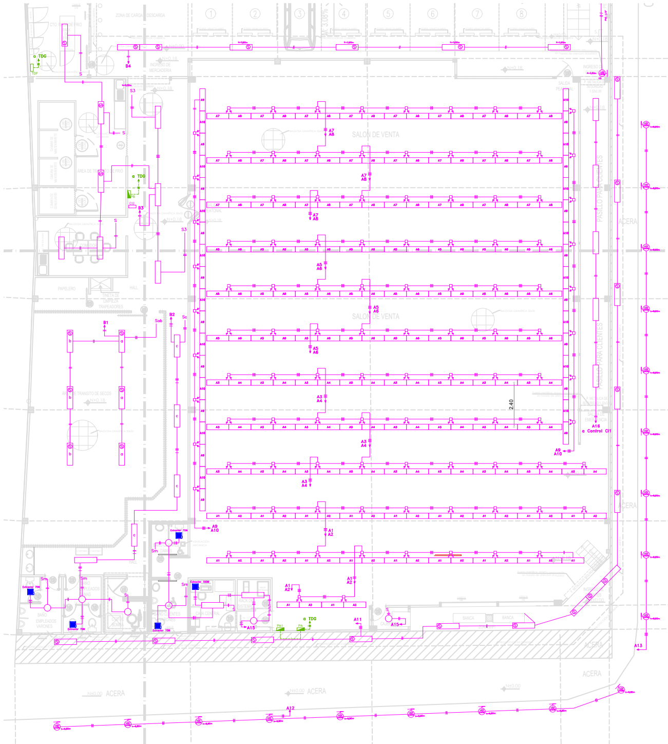
CIRCUITOS DE ALUMBRADO ESC_____1:75
