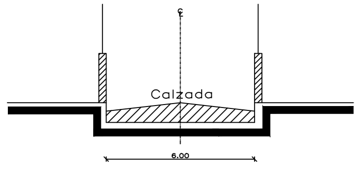
CORTE PASAJE S17D
