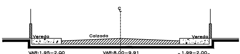
CORTE CALLE E12F CILLAHUA
