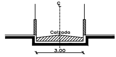
CORTE ESCALINATA E12E
