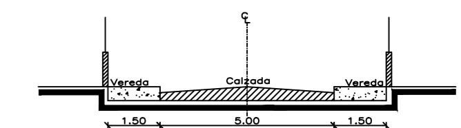
CORTE CALLE S18 Y E12C YAMTA
