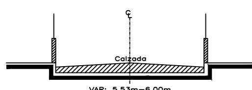
CORTE PASAJE S18A
