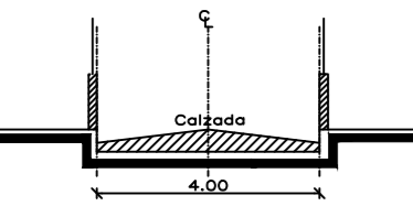
CORTE PASAJE E12G
