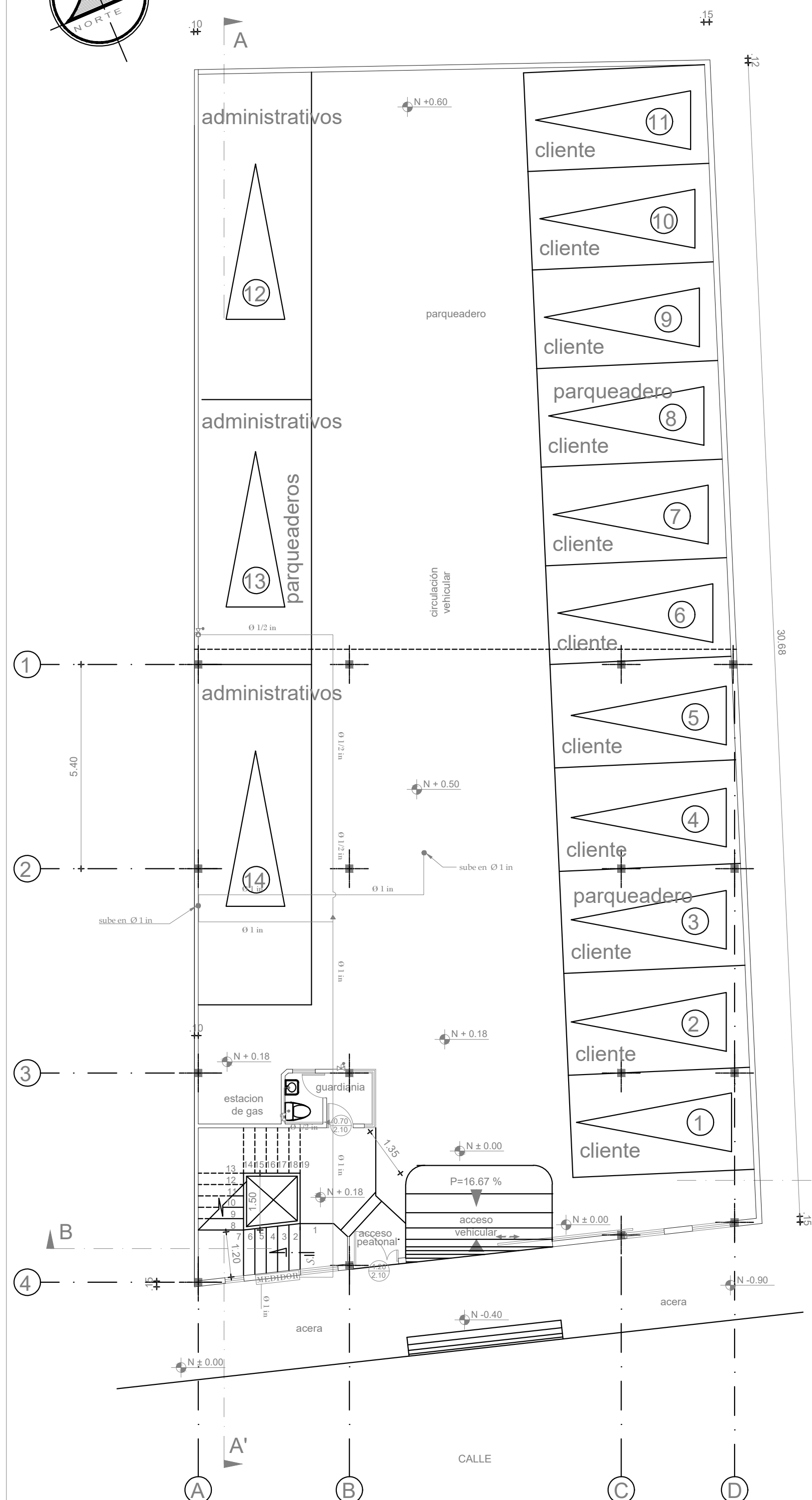
PLANTA BAJA Esc. 1:100
