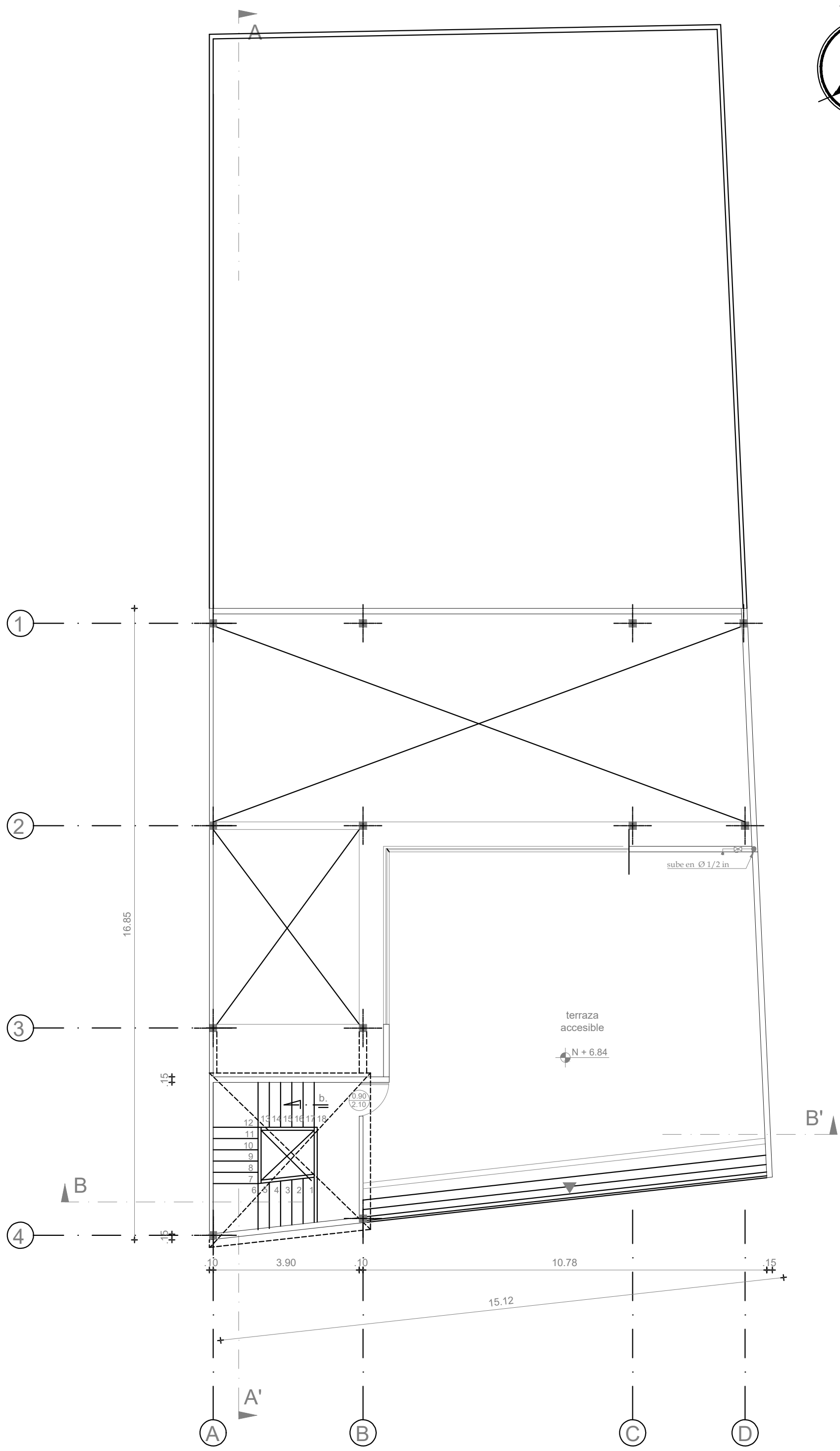
TERRAZA NIVEL +6.84 Esc. 1:100
