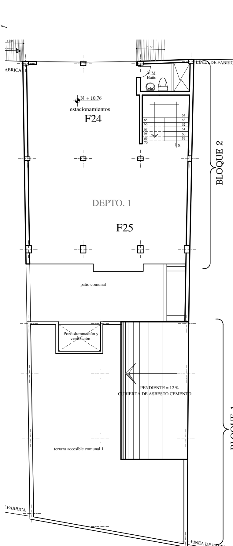
PLANTA ALTA BLOQUE 2 Escala :-----1:125
