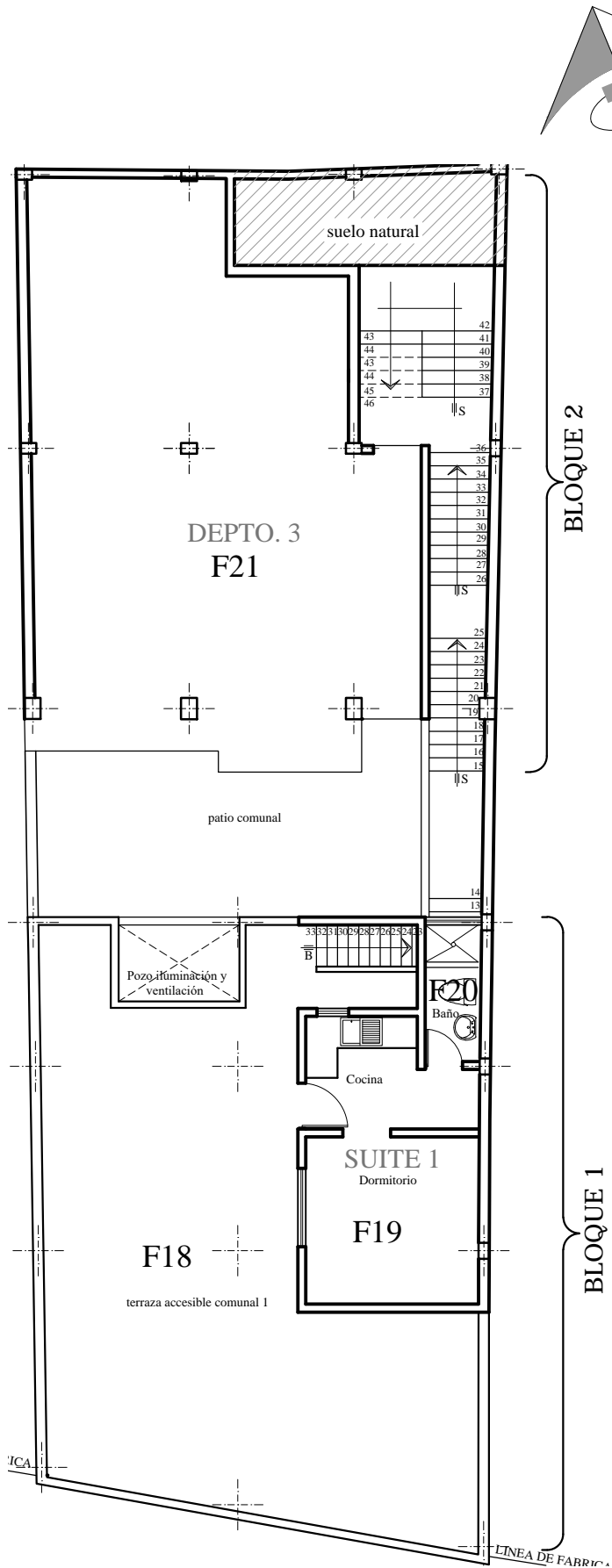
2DA PLANTA ALTA- BLOQUE 1 PLANTA BAJA- BLOQUE 2 SUBSUELO - BLOQUE 2 Escala :-----1:125
