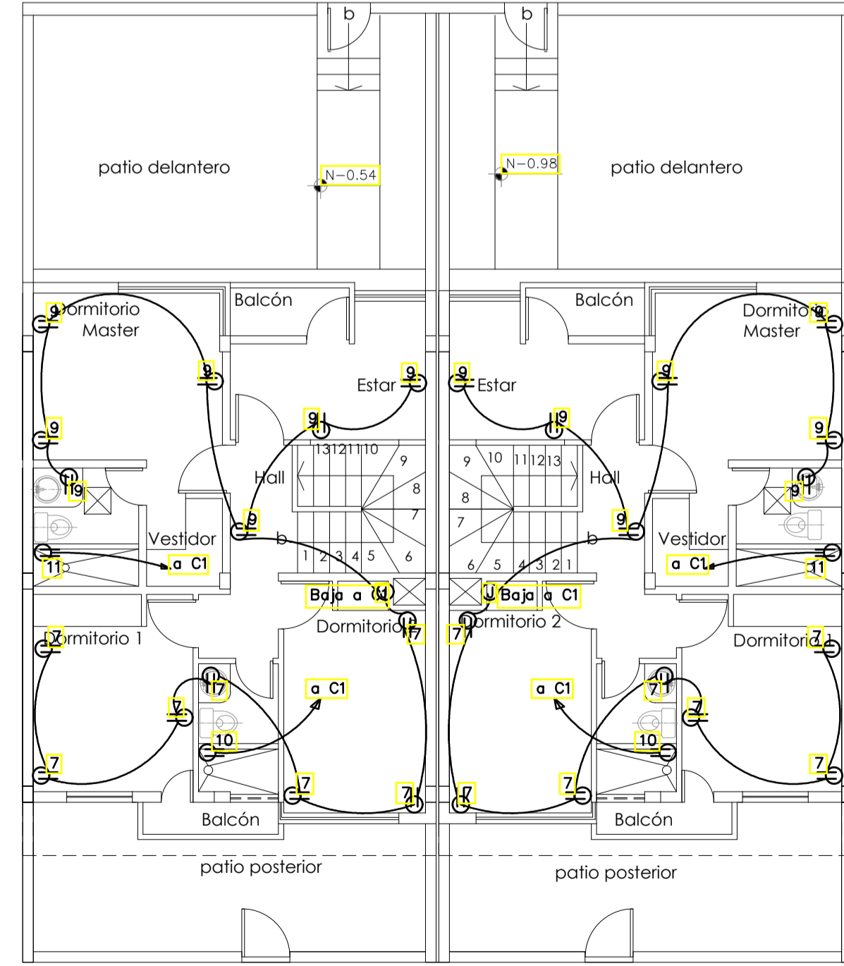
INSTALACIONES ELECTRICAS PLANTA ALTA CASA TIPO
