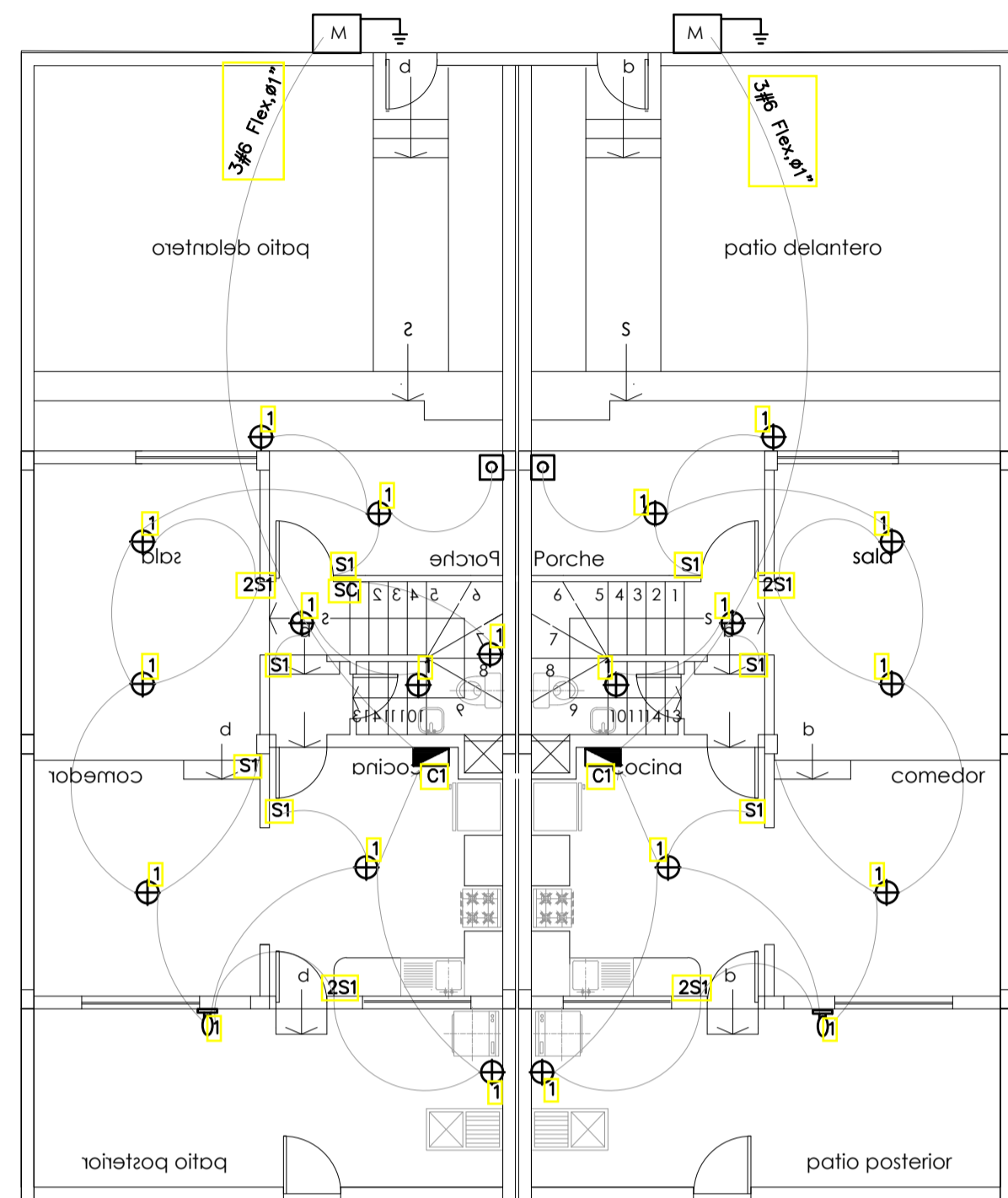
INSTALACIONES ELECTRICAS PLANTA BAJA CASA TIPO
