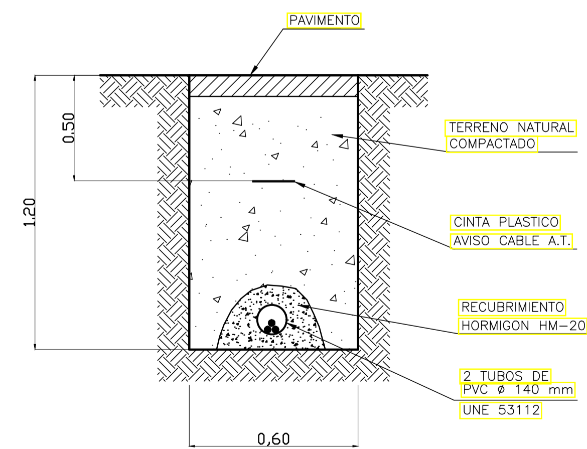
DETALLE ZANJA CABLE BAJO TUBO Escala: 1/20
