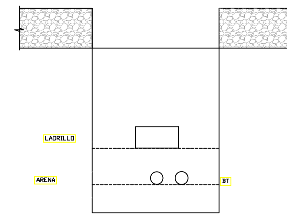
DETALLE CAJA BAJA TENSION
