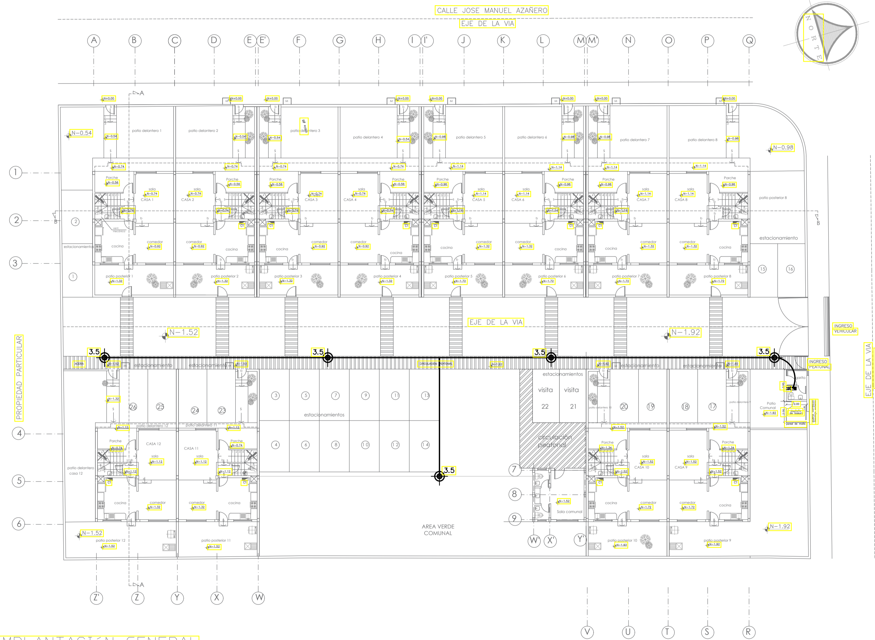
IMPLANTACIÓN GENERAL ESCALA 1=200
