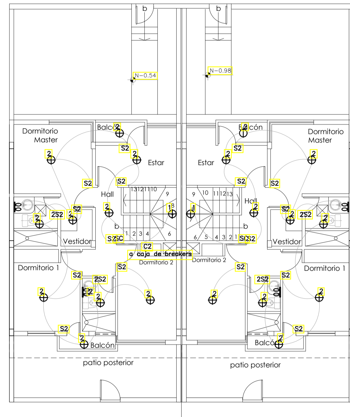
INSTALACIONES ELECTRICAS PLANTA ALTA CASA TIPO
