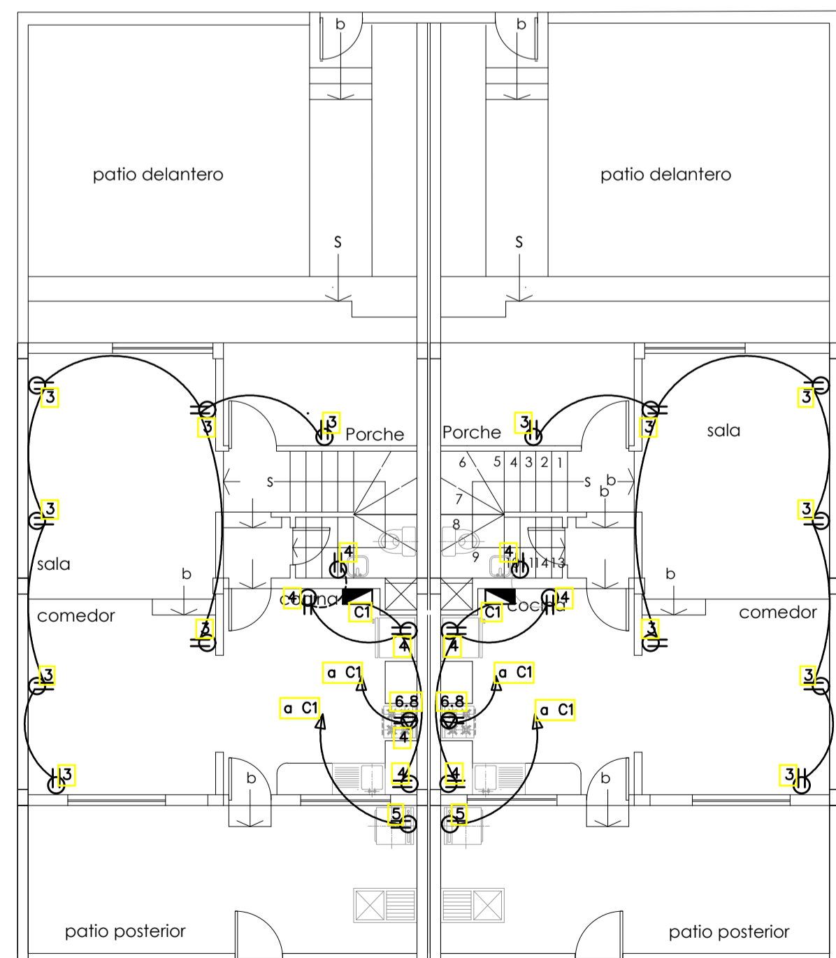
INSTALACIONES ELECTRICAS PLANTA BAJA CASA TIPO
