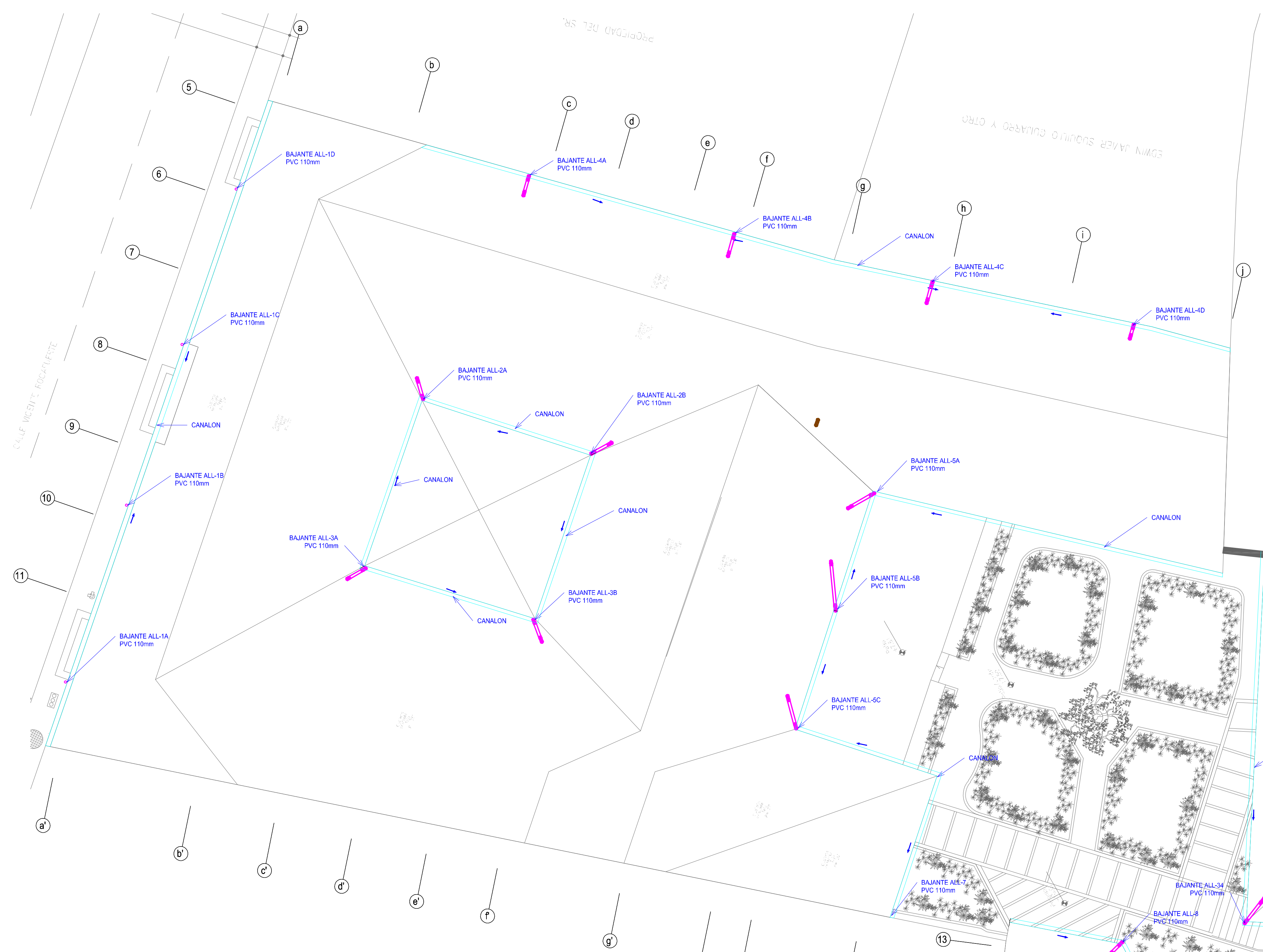
1 6.1 CUBIERTAS - SECTOR A ESC: 1:100
