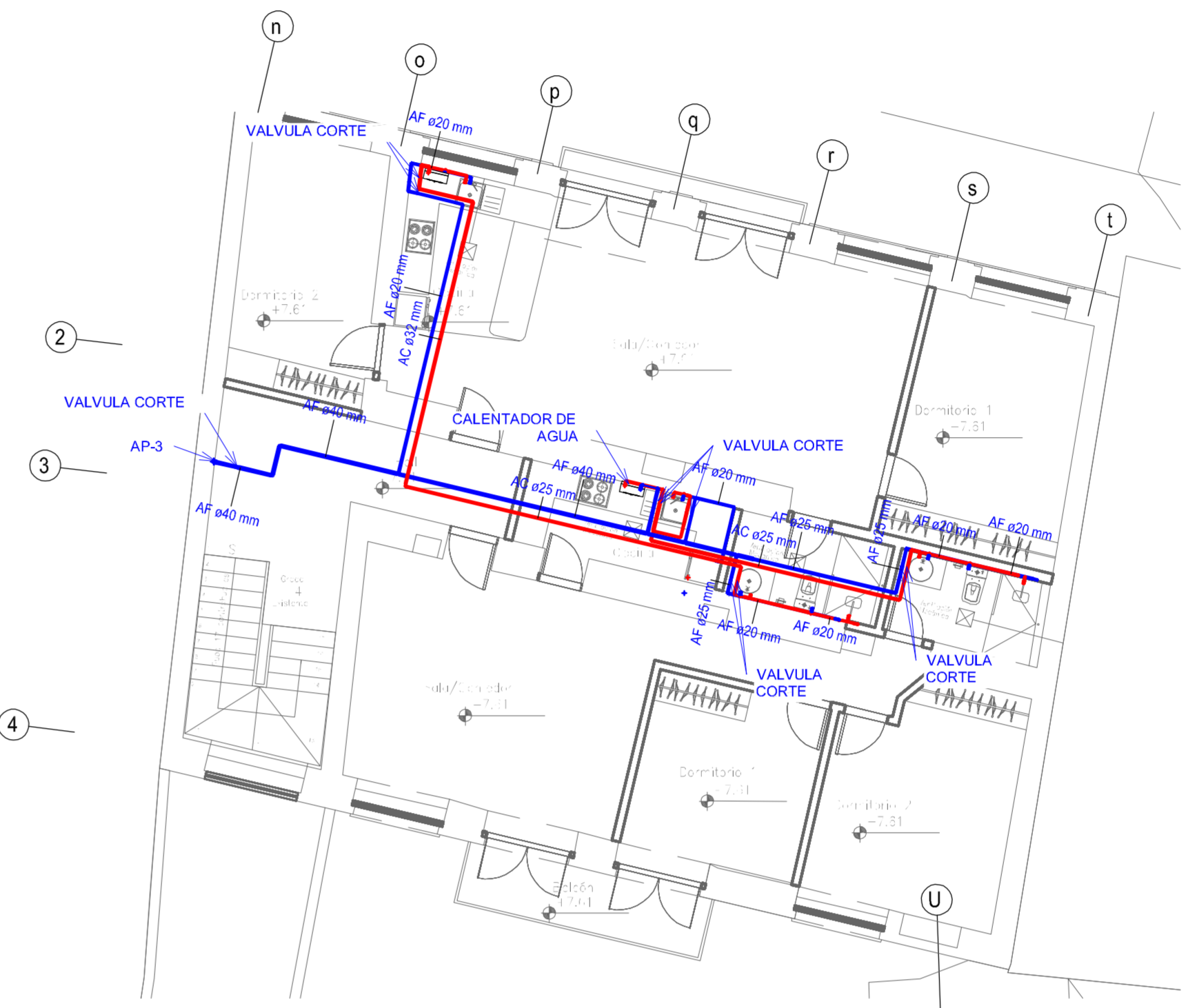
2 4.2 NIVEL +7.50 - SECTOR B 1:100
