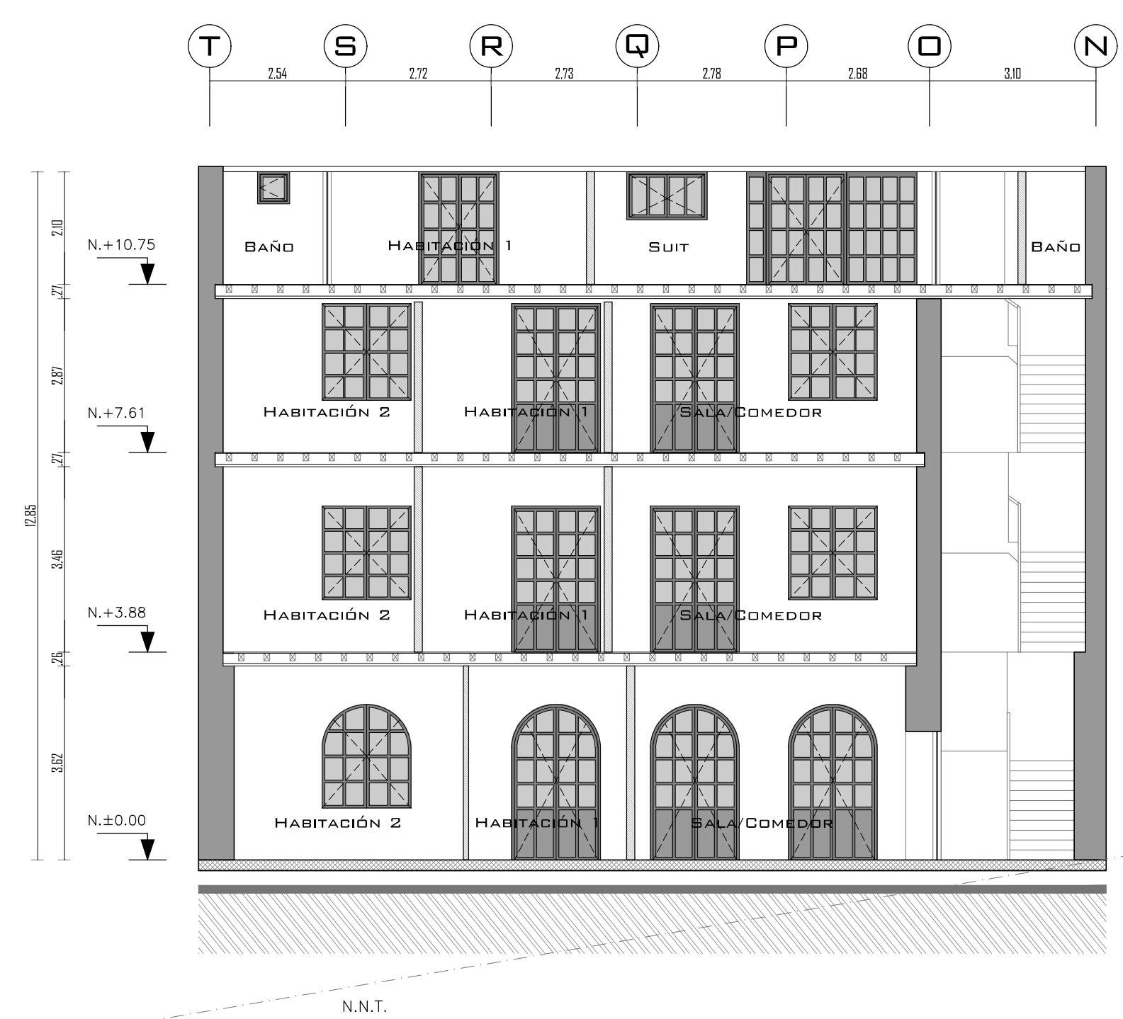
CORTE B-B 1 ESC: 1 _____ 100 0 1 2 3 4 5 6
