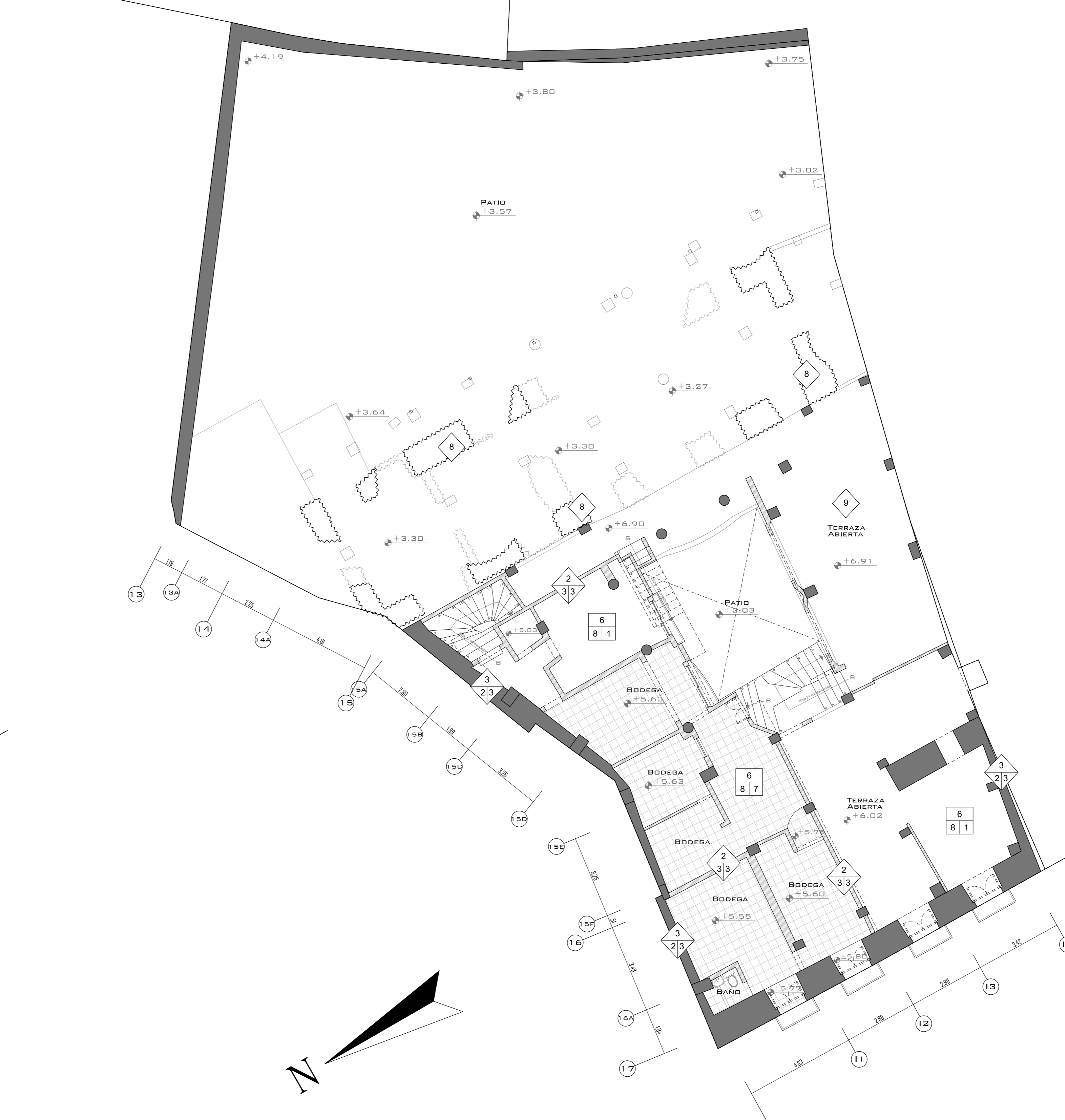
BLOQUE B PLANTA MATERIALES CONSTRUCTIVOS NIVEL +5.63/+6.91 ESC: 1 _____ 100 0 1 2 3 4 5 6
