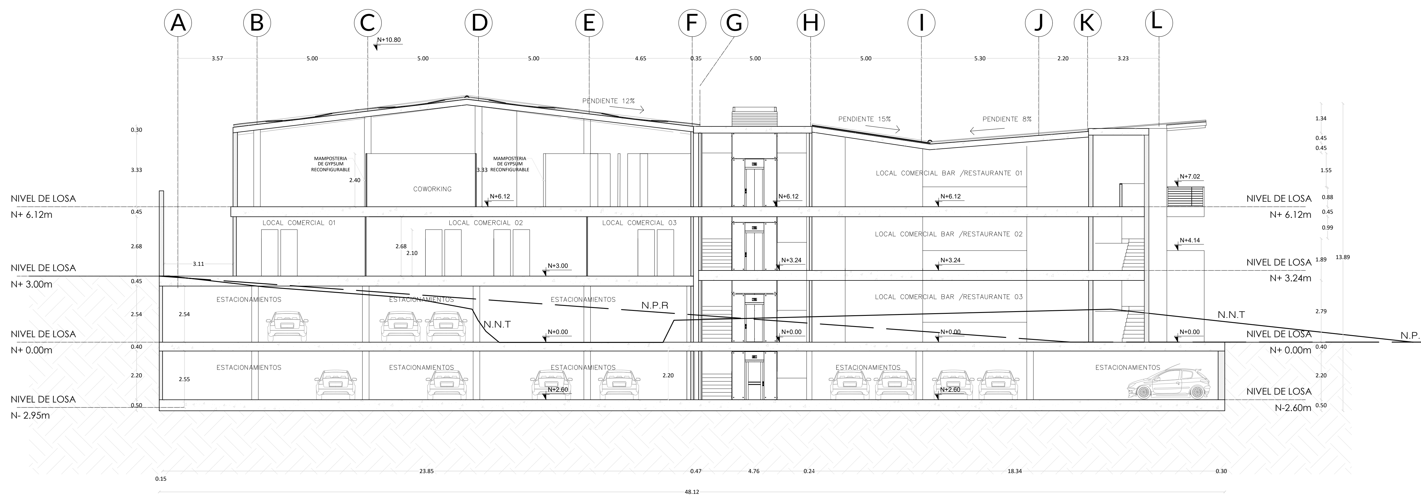
CORTE 1 - 1 ESC.: 1 100
